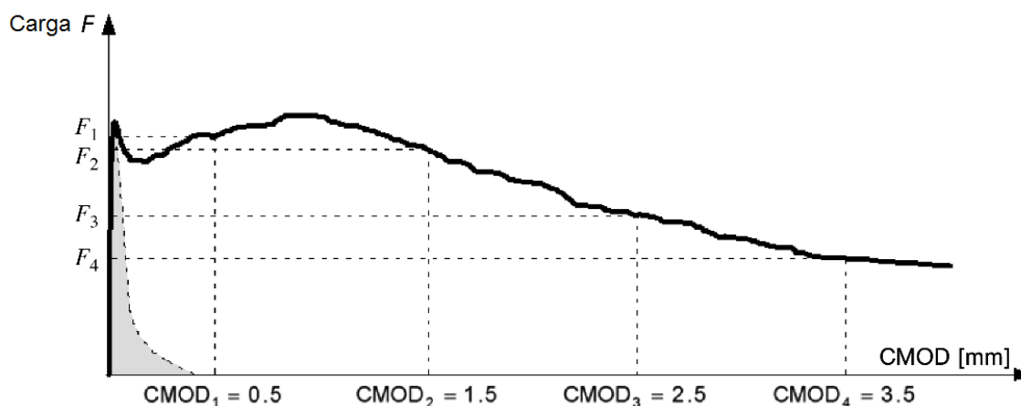
Figura 1 – Curva carga x CMOD
