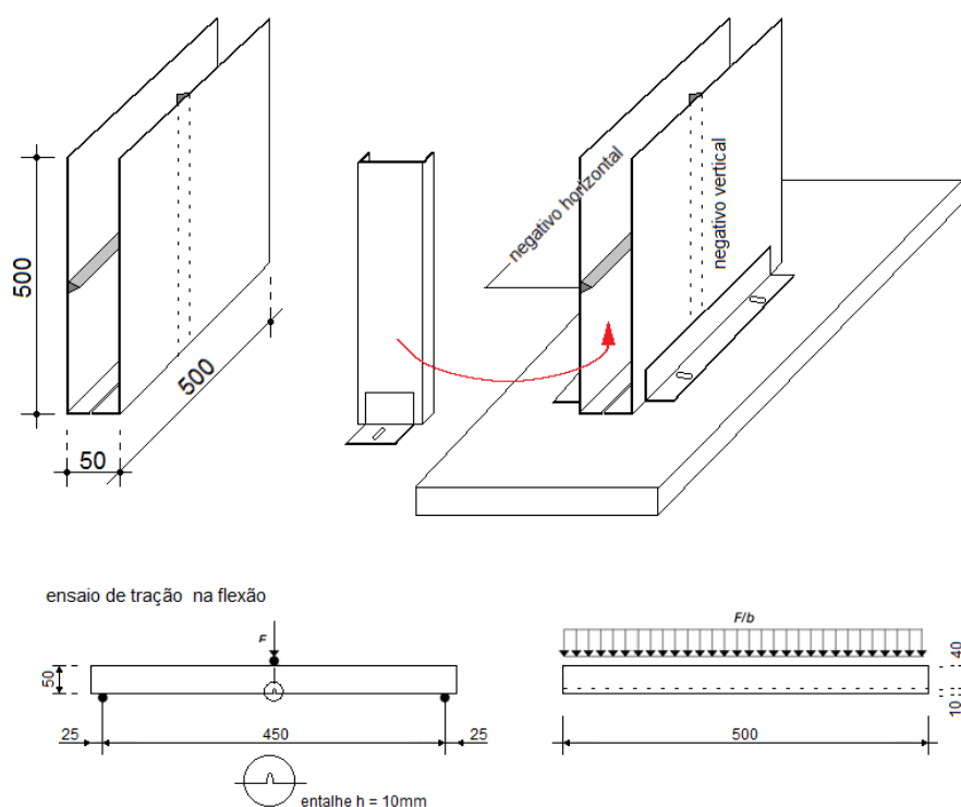
Figura 2 – Molde para corpos de prova 500x500x50 mm destinados à determinação da resistência à tração na flexão na direção do lançamento do concreto e na direção transversal
