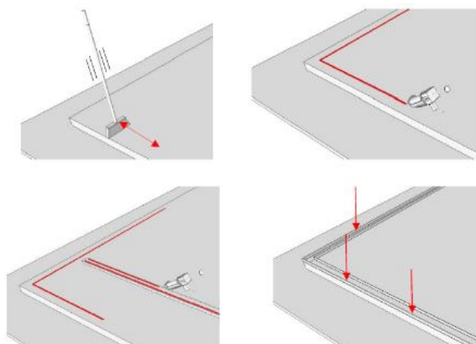
Figura 26 – Ilustração das etapas para posicionamento do perfil “BC 90” sobre o elemento de fundação (nesse caso do tipo radier ): 1º - limpeza do radier ; 2º - aplicação do cordão de selante na superfície do radier ; 3º - aplicação do cordão de selante na base do perfil “BC 90”; 4º - posicionamento do perfil “BC 90” sobre o radier . (Sem escala).
