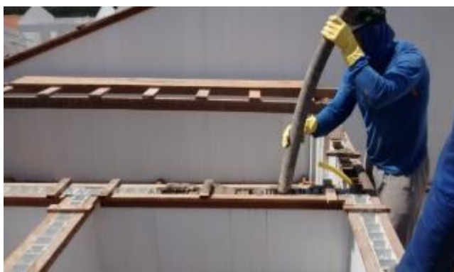
Figura 76 – Lançamento do concreto autoadensável no interior dos painéis de PVC rígido (travados com as guias de topo).
