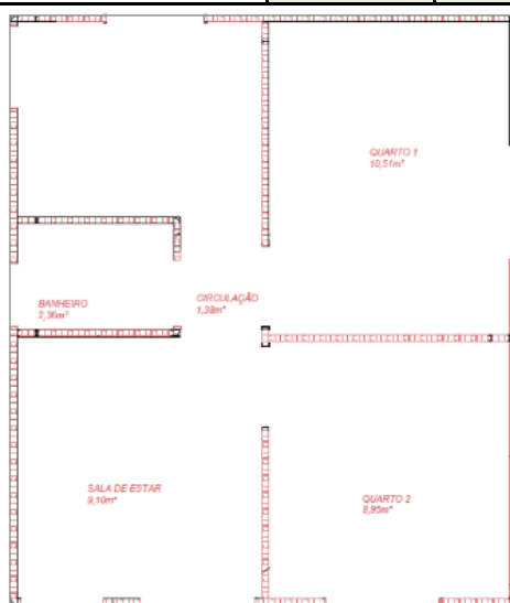
Figura 92 – Planta do protótipo do Sistema Construtivo Basse PVC objeto dos ensaios para avaliação do desempenho acústico em campo.
