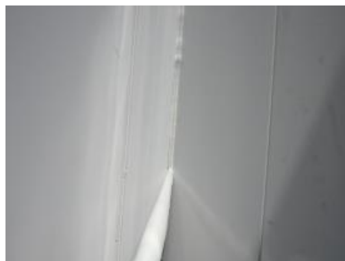
Figura 73 – Preenchimento das juntas entre as paredes perpendiculares com selante poliuretano monocomponente.
