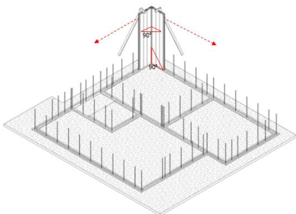
Figura 58 – Ilustração do início da montagem dos painéis pelos vértices das paredes externas.
