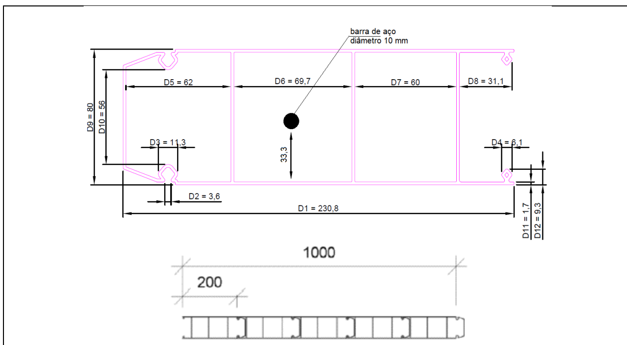
Figura 6 – Ilustração do perfil “BC 200” com barra de armadura inserida e exemplo de modulação básica de parede montada com perfis “BC 200”. (Dimensões em milímetros - sem escala).
