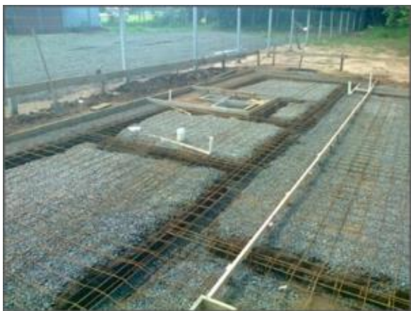
Figura 53 – Localização das armaduras da fundação e das tubulações que ficarão sob o elemento de fundação (nesse caso radier ).
