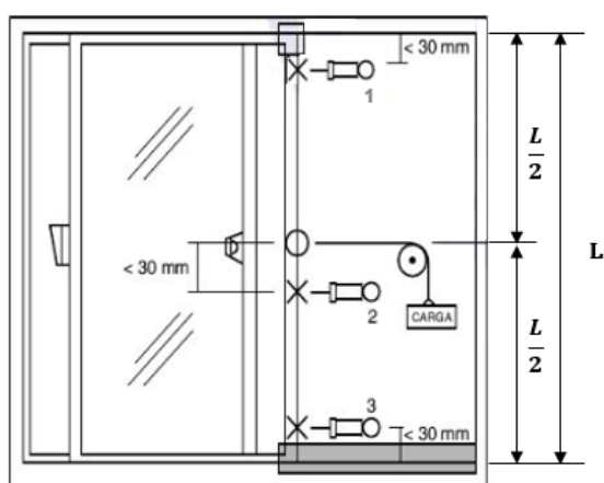
Figura 15 – Esquema de Posicionamento dos Relógios Comparadores (Esquerda) e Execução do Ensaio (Direita)
