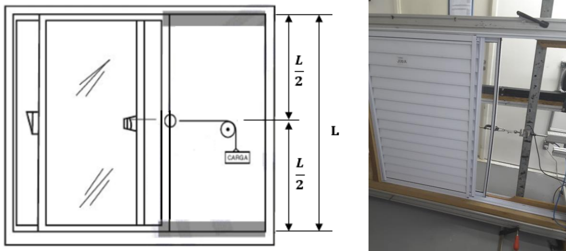
Figura 16 – Esquema do Ensaio Para Esquadrias de Correr (Esquerda) e Execução do Ensaio (Direita)
