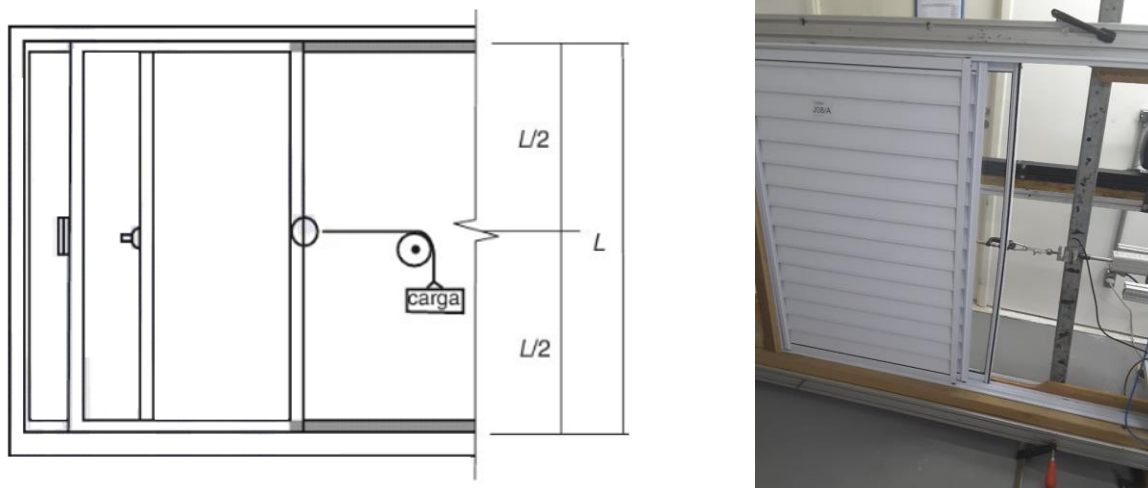
Figura 7 – Esquema do ensaio para esquadrias de correr (esquerda) e execução do ensaio (direita)
