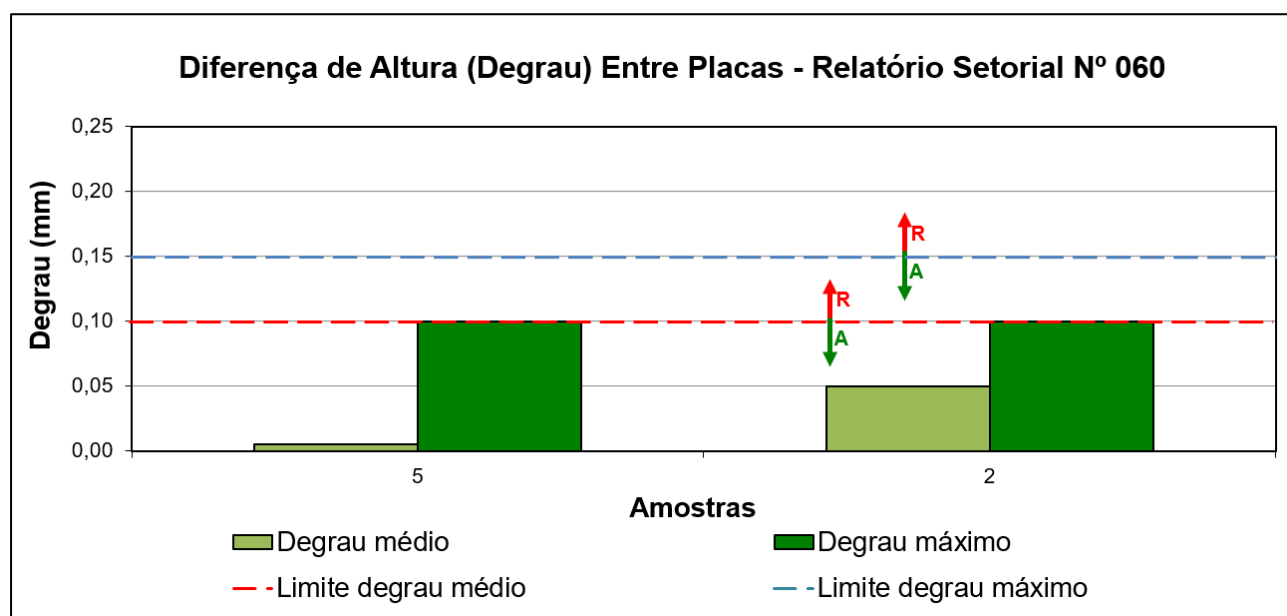
Figura 7 - Resultados obtidos no ensaio de determinação da diferença de altura (degrau) entre placas em pisos laminados melamínicos de classe de abrasão AC3 e AC4 produzidos por empresas participantes
