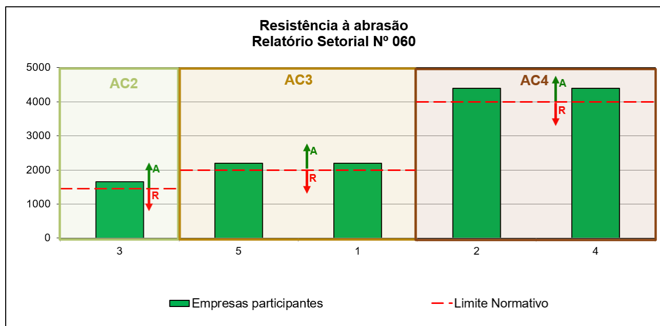
Figura 5 - Resultados obtidos no ensaio de determinação da resistência à abrasão em pisos laminados melamínicos de classe de abrasão AC2, AC3 e AC4 produzidos por empresas participantes
