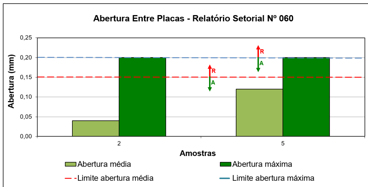
Figura 6 - Resultados obtidos no ensaio de determinação da abertura entre placas em pisos laminados melamínicos de classe de abrasão AC3 e AC4 produzidos por empresas participantes
