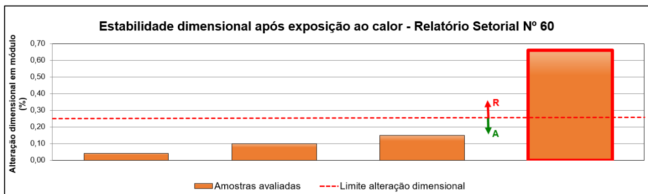
Figura 12 - Resultados obtidos no ensaio de determinação da estabilidade dimensional após exposição ao calor em pisos laminados vinílicos produzidos por empresas participantes e não participantes
