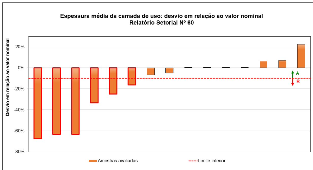
Figura 9 - Resultados obtidos no ensaio de determinação da espessura nominal média da camada de uso em pisos laminados vinílicos produzidos por empresas participantes e não participantes
