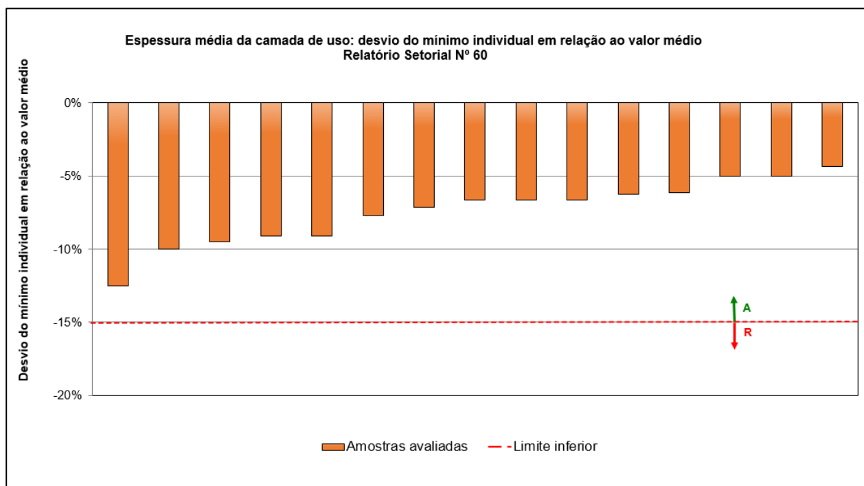
Figura 10 - Resultados obtidos no ensaio de determinação da espessura nominal média da camada de uso em pisos laminados vinílicos produzidos por empresas participantes e não participantes
