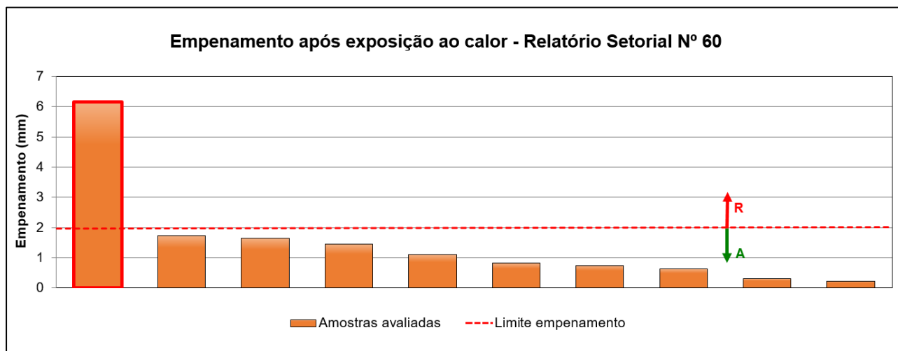
Figura 11 - Resultados obtidos no ensaio de determinação do empenamento após exposição ao calor em pisos laminados vinílicos produzidos por empresas participantes e não participantes
