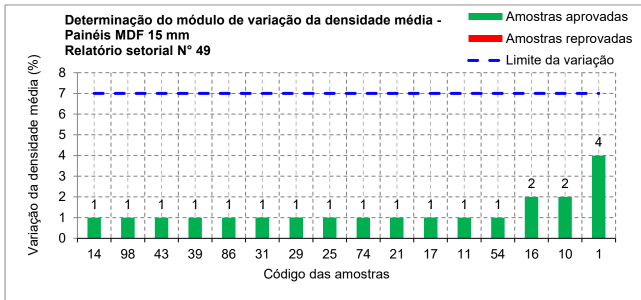
Figura 7 – Determinação do módulo de variação da densidade média de painéis MDF com espessura igual a 15 mm
