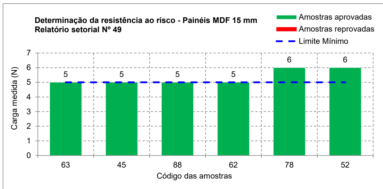
Figura 8 – Determinação da resistência ao risco de painéis MDF com revestimento BP, nas duas faces, de 15 mm de espessura
