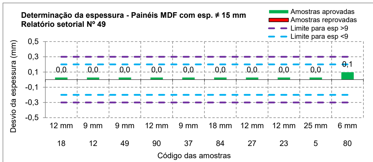
Figura 4 - Determinação do desvio da espessura de painéis MDF com espessura diferente de 15 mm
