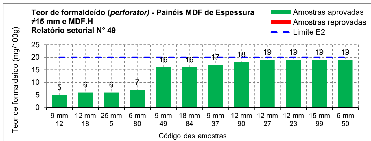
Figura 3 - Teor de formaldeído (método perforator ) de painéis MDF sem revestimento de espessuras diferentes de 15 mm e painéis MDF.H de todas as espessuras
