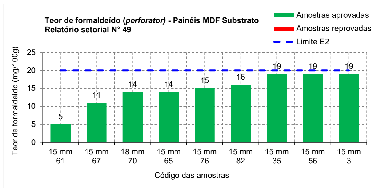
Figura 10 - Teor de formaldeído (método perforator ) de chapas de MDF utilizadas na fabricação de painéis revestidos
