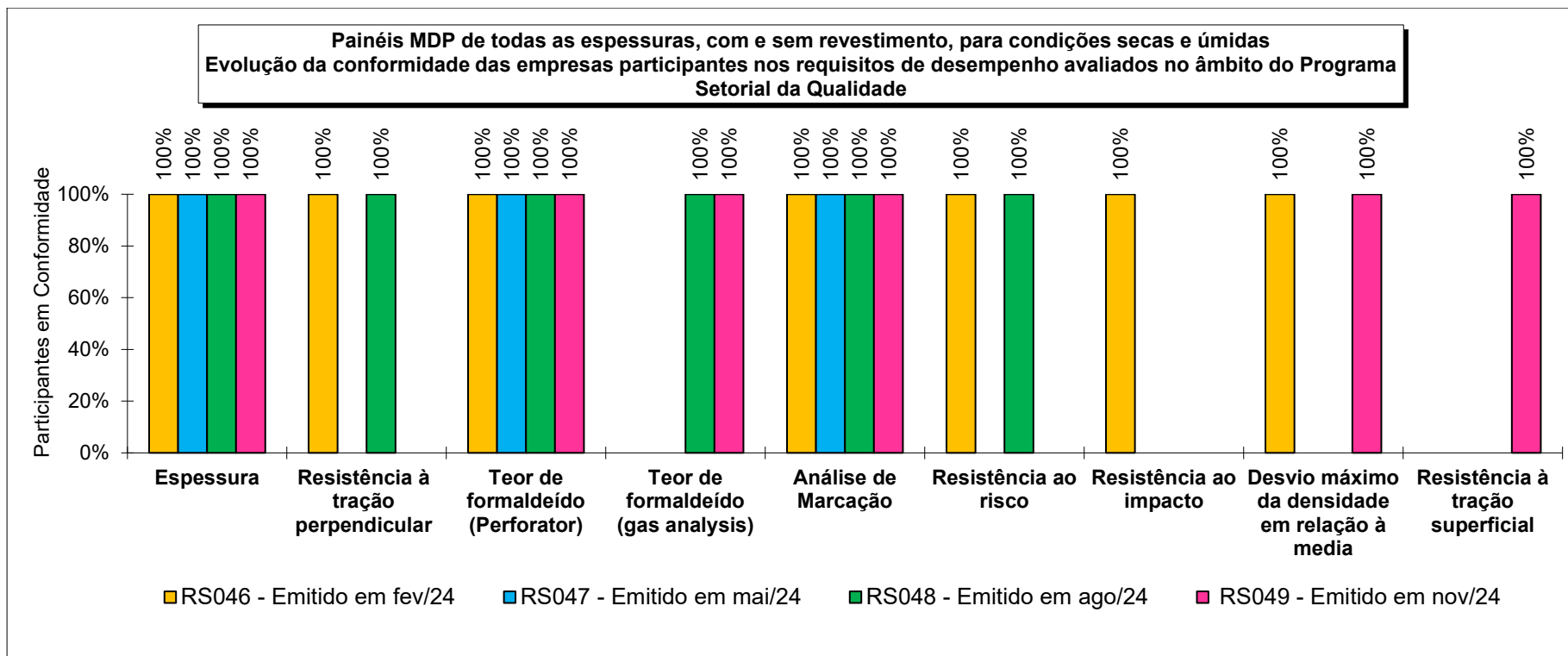
Figura 21 - Evolução da conformidade das empresas participantes nos requisitos de desempenho aplicáveis a painéis MDP de todas as espessuras, com e sem revestimento, para uso geral (não estrutural) em condições secas e condições úmidas, e avaliados no âmbito do Programa Setorial da Qualidade.
