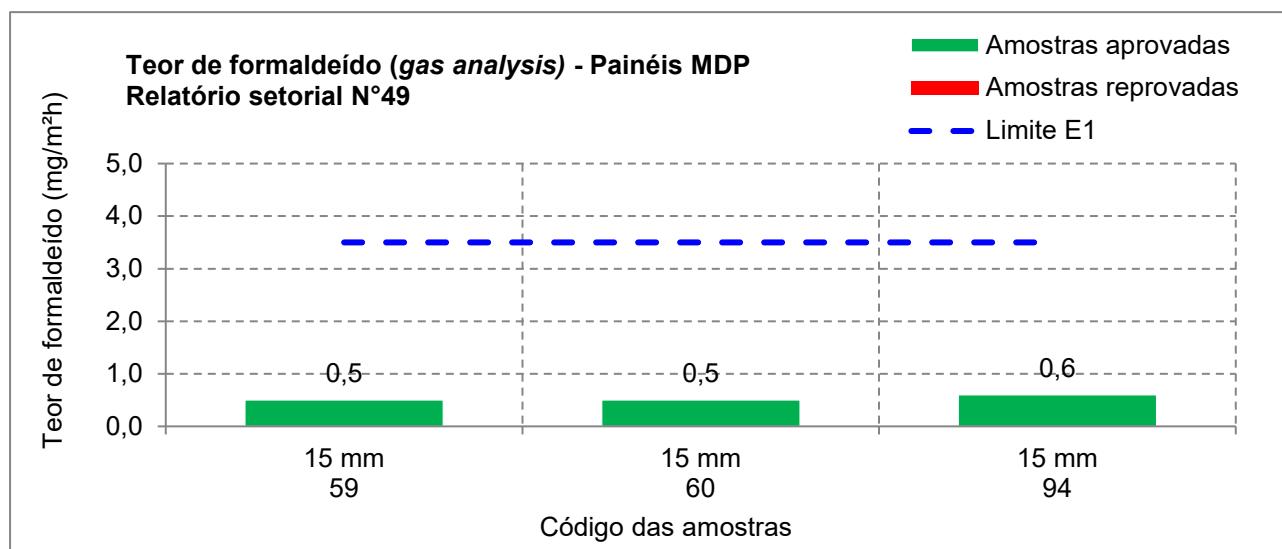
Figura 17 - Determinação de formaldeído (método gas analysis ) de painéis MDP com revestimento BP, nas duas faces, de espessura iguais a 15 mm
