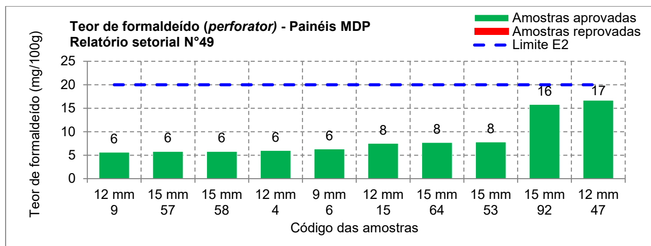
Figura 11 - Teor de formaldeído (método perforator ) de painéis MDP sem revestimento de espessura de 15 mm e diferente de 15 mm
