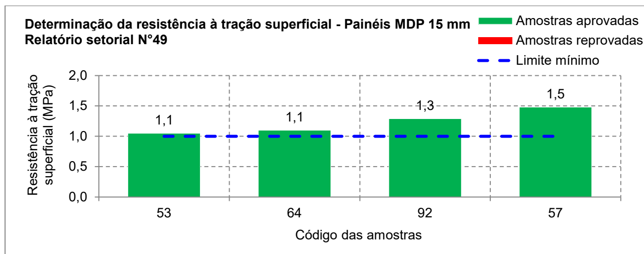
Figura 14 - Determinação da resistência à tração superficial de painéis MDP com espessura de 15 mm
