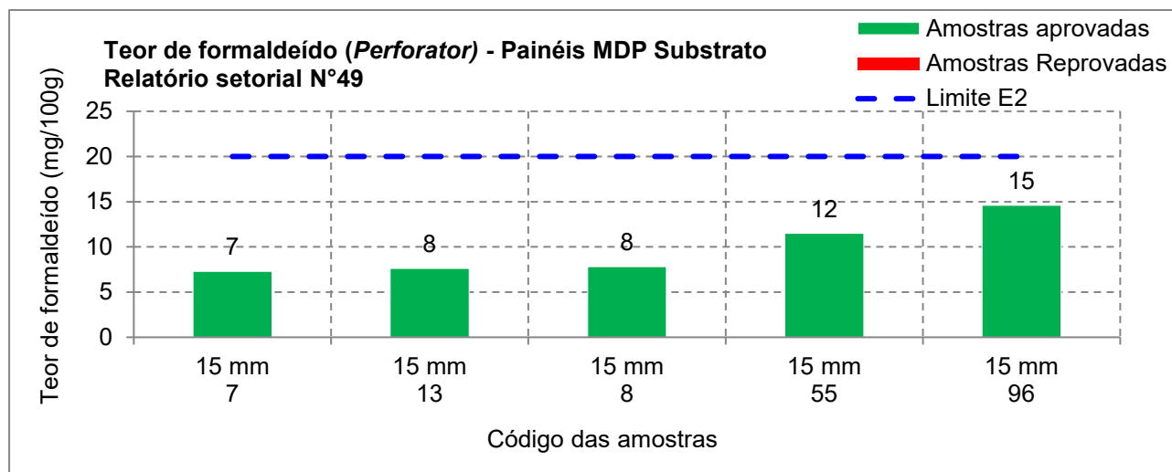
Figura 19 - Teor de formaldeído (método perforator ) de chapas de MDP utilizadas na fabricação de painéis revestidos
