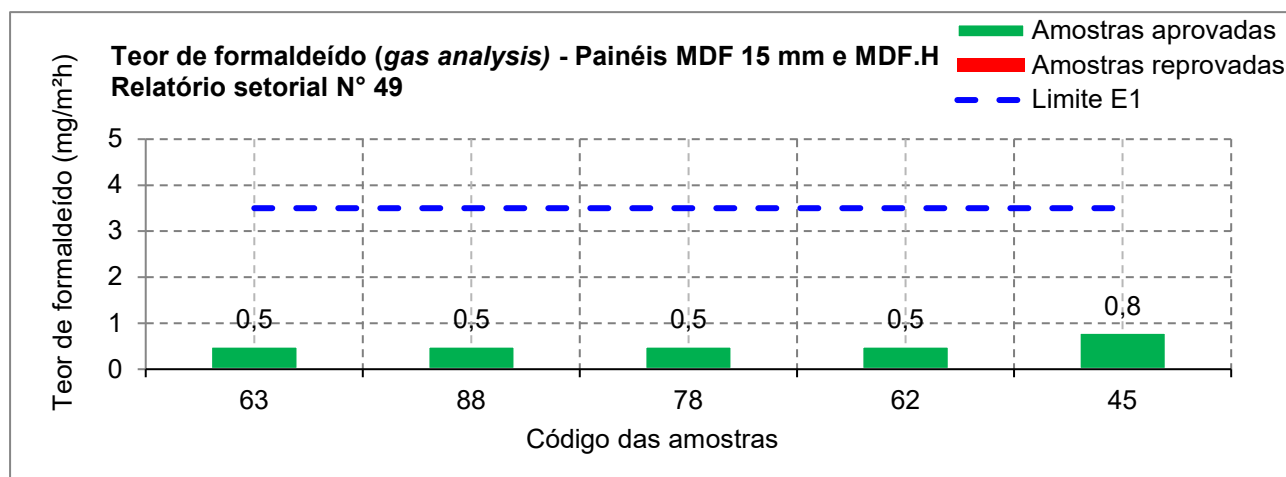
Figura 9 – Determinação de formaldeído (método gas analysis ) de painéis MDF com revestimento BP, nas duas faces, de espessura iguais a 15 mm
