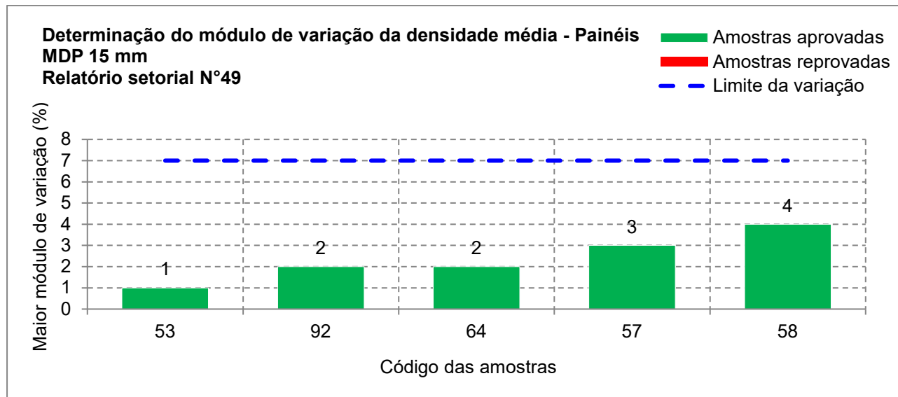
Figura 15 - Determinação do módulo de variação da densidade média de painéis MDP com espessura igual a 15 mm
