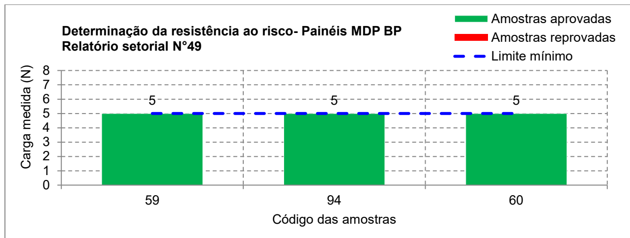
Figura 16 – Determinação da resistência ao risco de painéis MDP com revestimento BP, nas duas faces, de 15 mm de espessura
