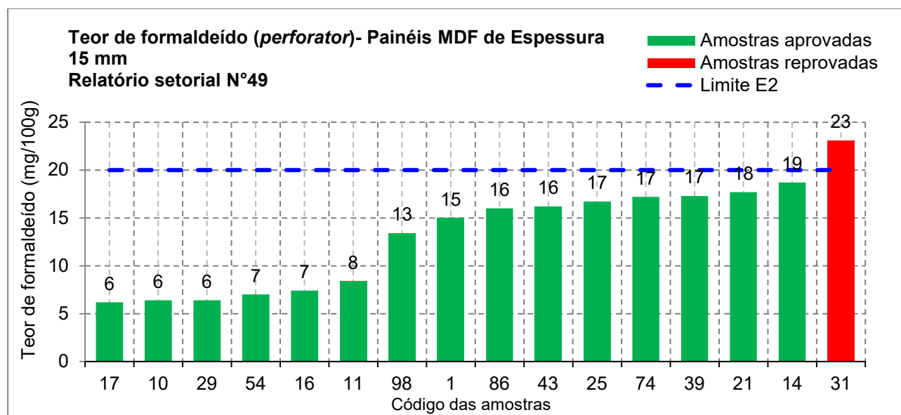
Figura 2 - Teor de formaldeído (método perforator ) de painéis MDF sem revestimento de 15 mm de espessura
