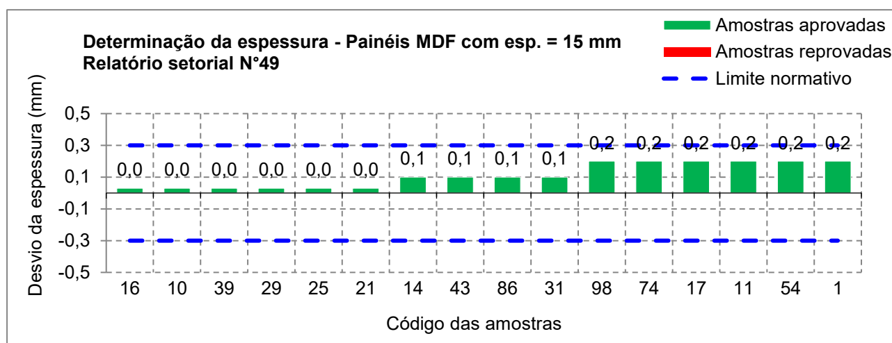
Figura 5 - Determinação do desvio de espessura de painéis MDF com espessura igual a 15 mm
