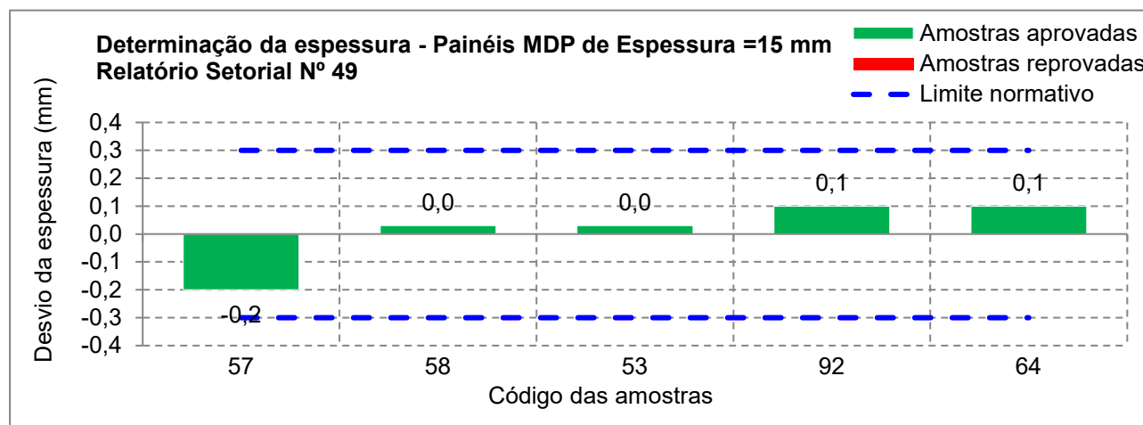
Figura 12 - Determinação do desvio de espessura de painéis MDP com espessura igual a 15 mm
