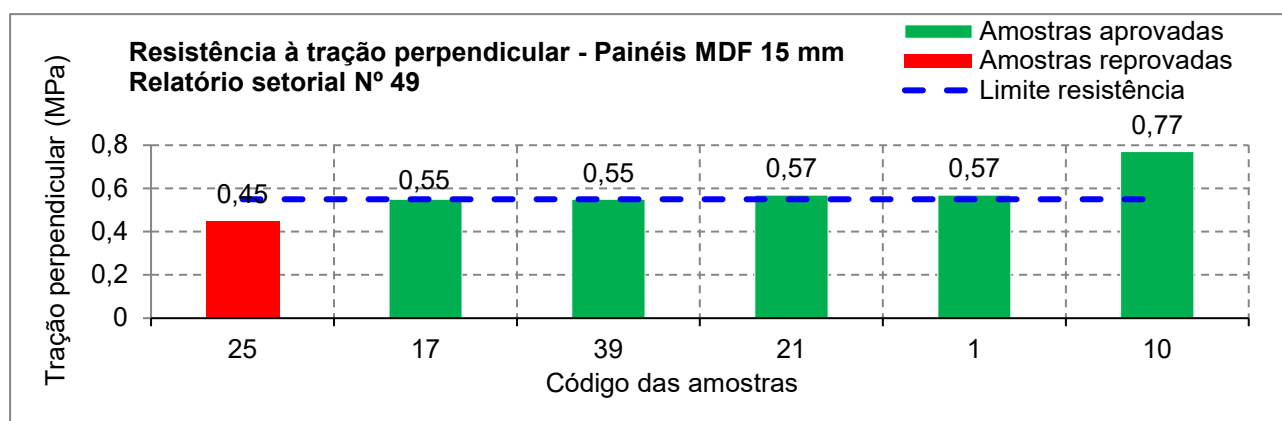
Figura 6 - Resistência à tração perpendicular de painéis MDF sem revestimento de 15 mm de espessura
