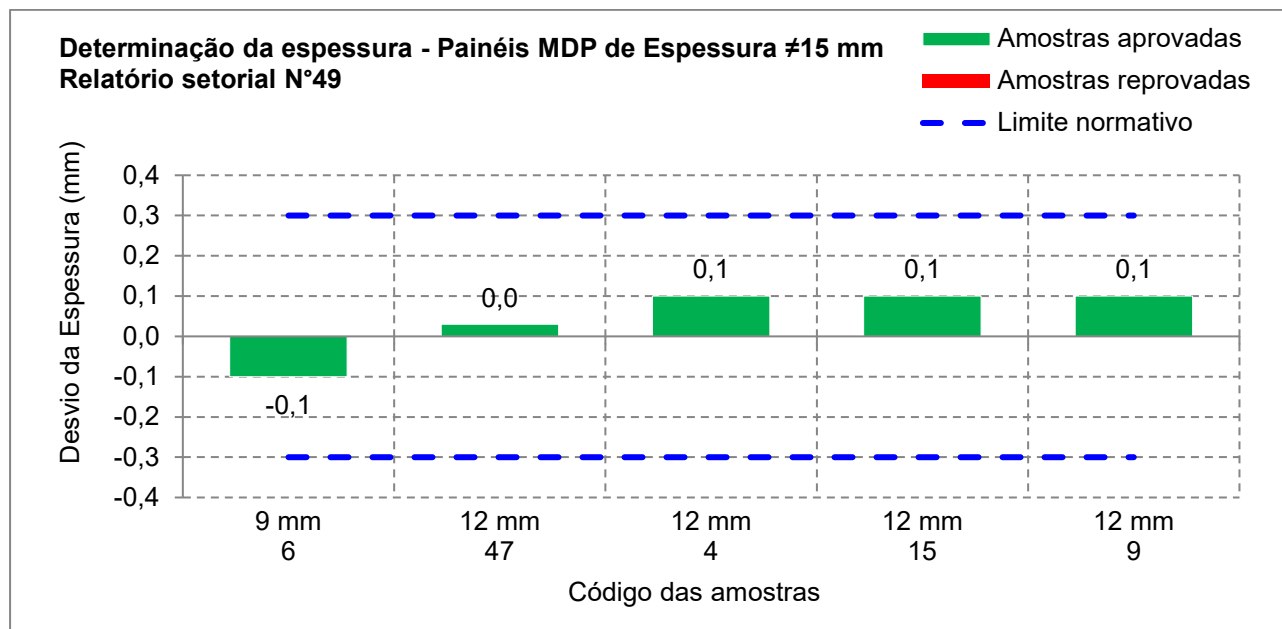
Figura 13 - Determinação do desvio de espessura de painéis MDP com espessura diferente de 15 mm
