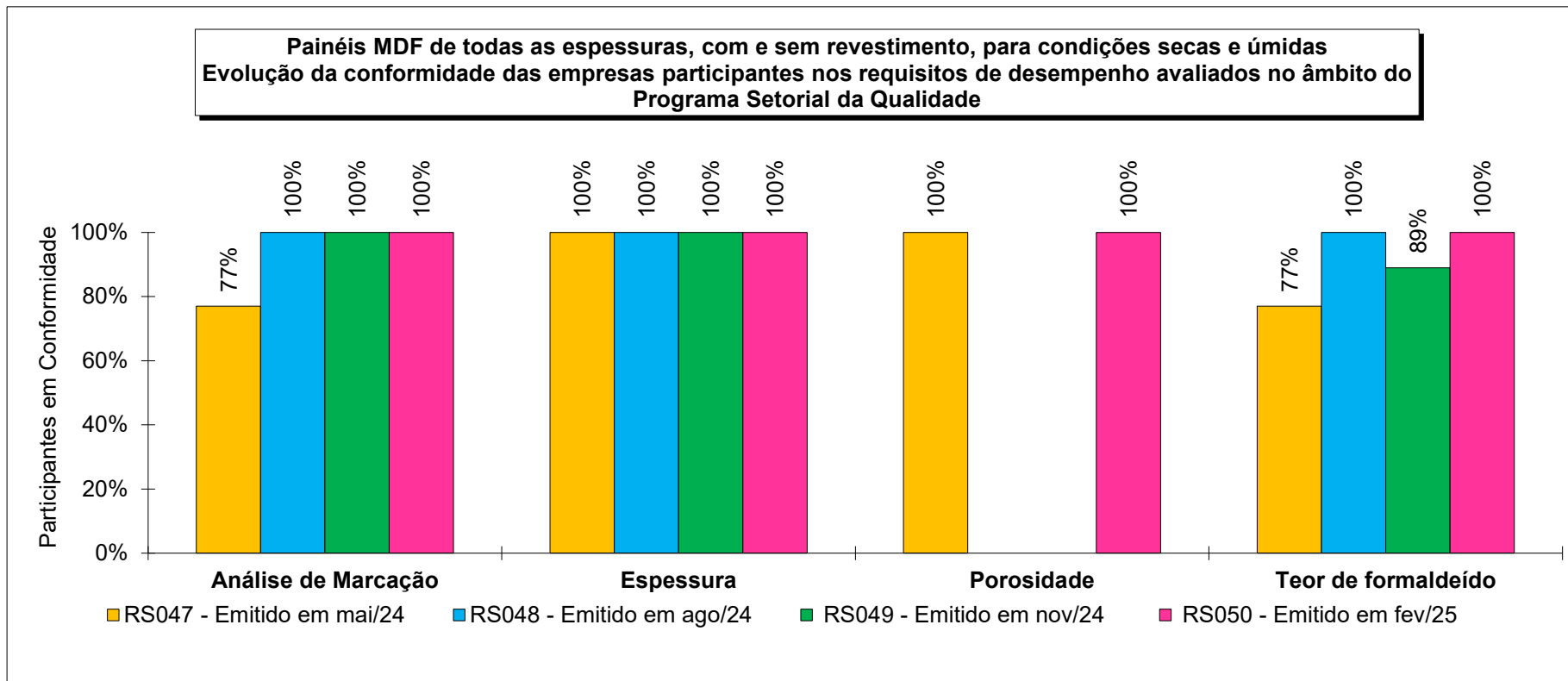
Figura 13- Evolução da conformidade das empresas participantes nos requisitos de desempenho aplicáveis a painéis MDF de todas as espessuras, com e sem revestimento, para uso geral (não estrutural) em condições secas e condições úmidas, e avaliados no âmbito do Programa Setorial da Qualidade
