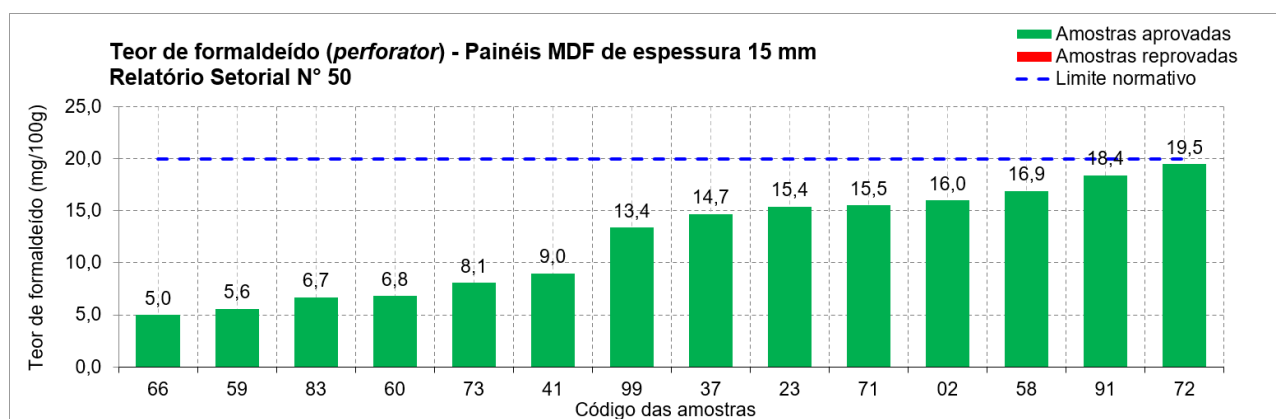
Figura 2 - Teor de formaldeído (método perforator ) de painéis MDF sem revestimento de 15 mm de espessura
