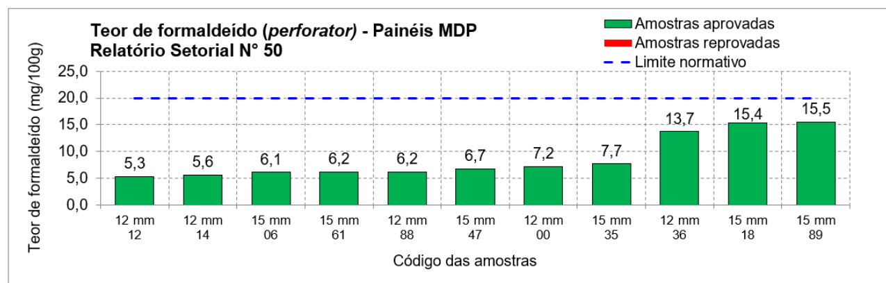
Figura 8 - Teor de formaldeído (método perforator ) de painéis MDP sem revestimento de espessura de 15 mm e diferente de 15 mm
