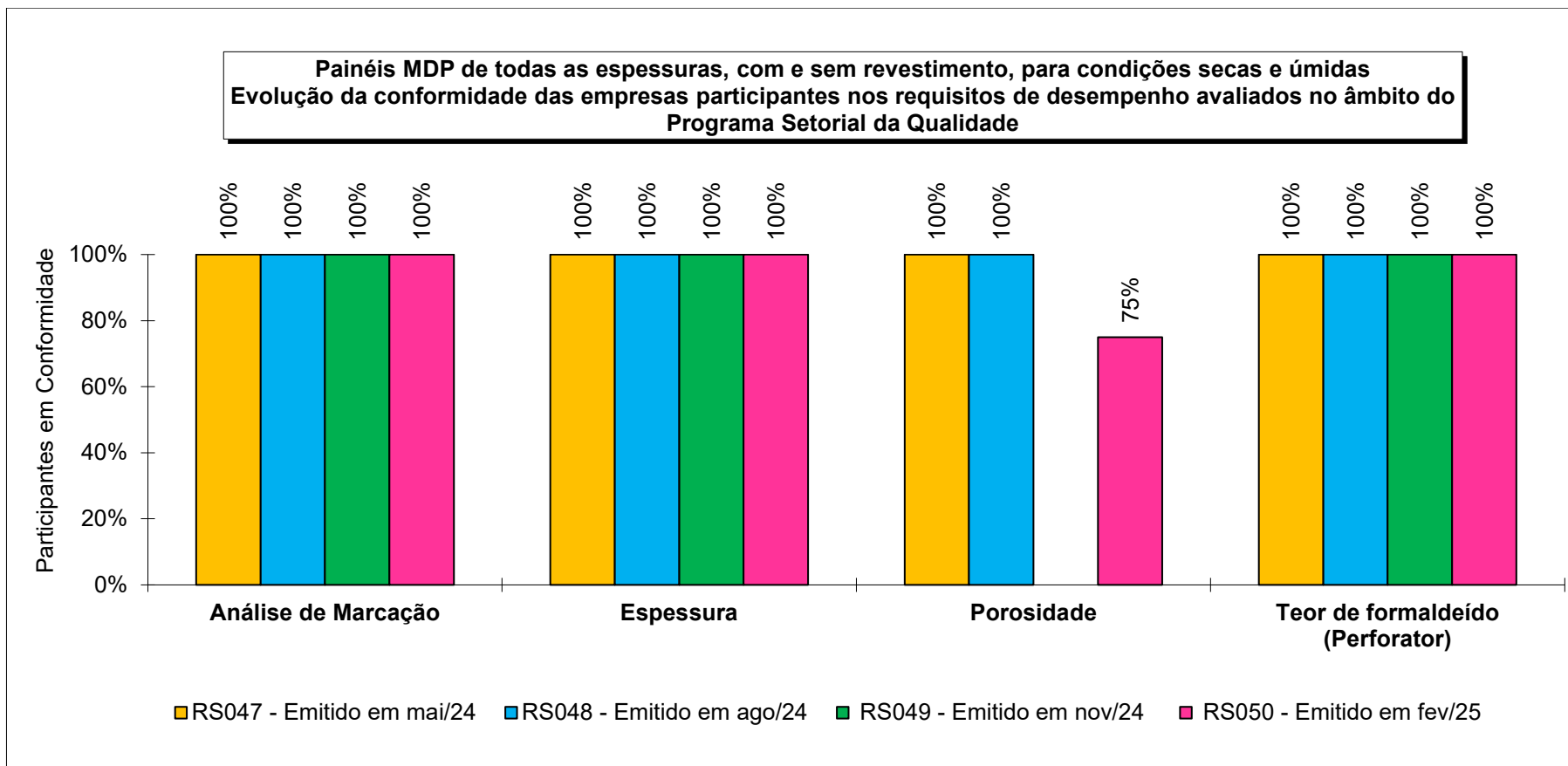
Figura 14 - Evolução da conformidade das empresas participantes nos requisitos de desempenho aplicáveis a painéis MDP de todas as espessuras, com e sem revestimento, para uso geral (não estrutural) em condições secas e condições úmidas, e avaliados no âmbito do Programa Setorial da Qualidade.
