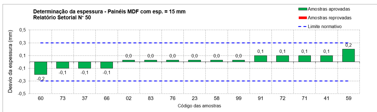
Figura 5 - Determinação do desvio de espessura de painéis MDF com espessura igual a 15 mm
