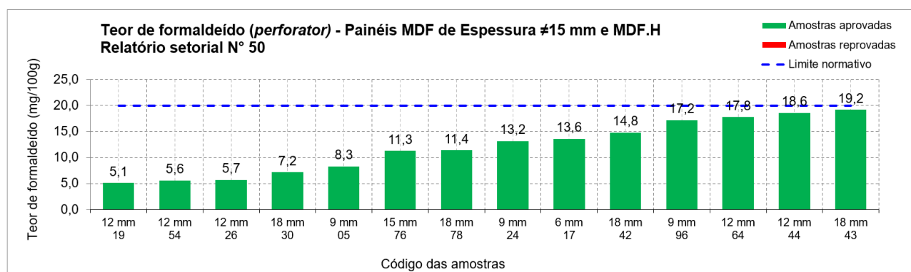
Figura 3 - Teor de formaldeído (método perforator ) de painéis MDF sem revestimento de espessuras diferentes de 15 mm e painéis MDF.H de todas as espessuras
