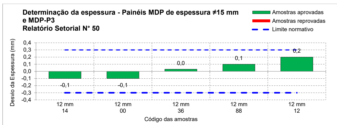
Figura 10 - Determinação do desvio de espessura de painéis MDP com espessura diferente de 15 mm
