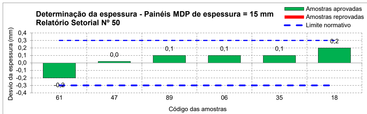
Figura 9 - Determinação do desvio de espessura de painéis MDP com espessura igual a 15 mm
