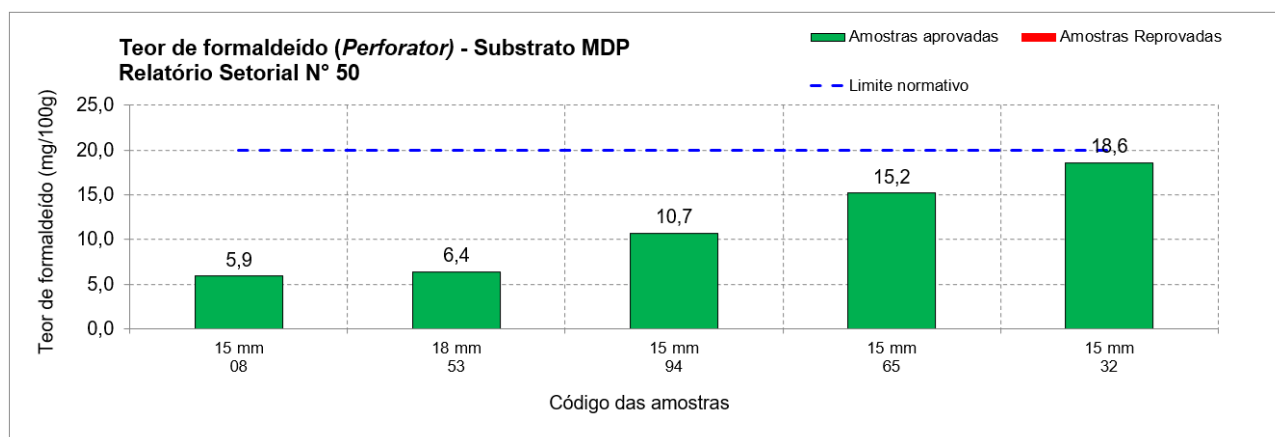
Figura 12 - Teor de formaldeído (método perforator ) de chapas de MDP utilizadas na fabricação de painéis revestidos
