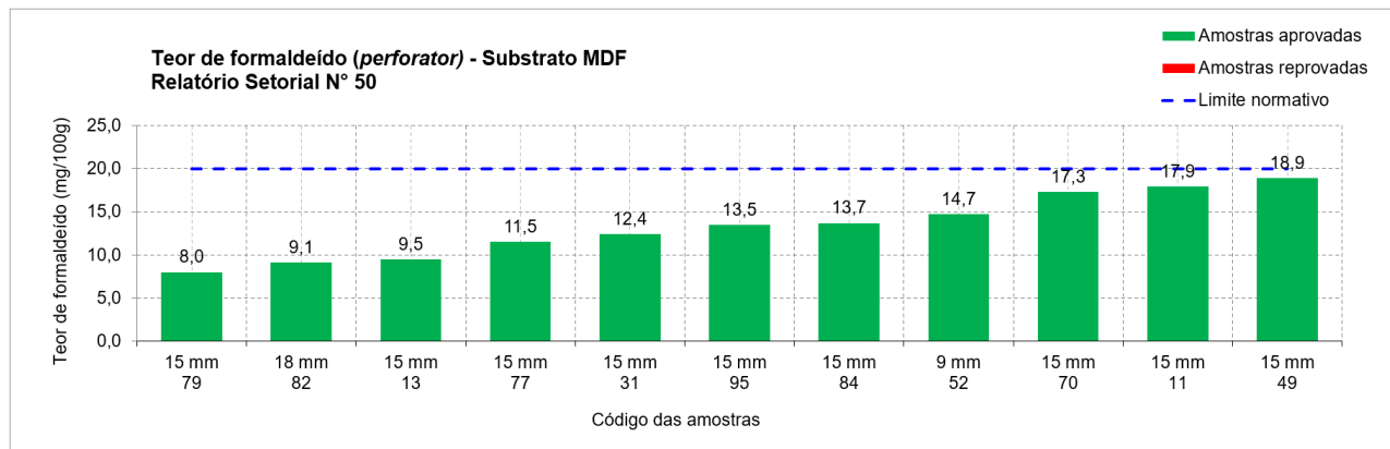
Figura 7 - Teor de formaldeído (método perforator ) de chapas de MDF utilizadas na fabricação de painéis revestidos
