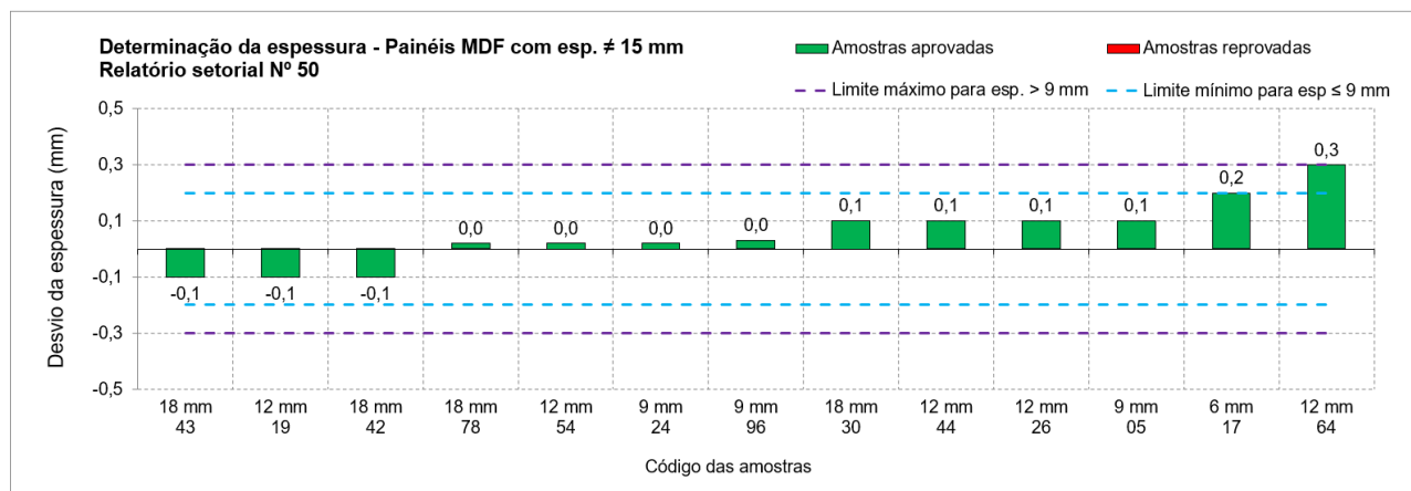
Figura 4 - Determinação do desvio da espessura de painéis MDF com espessura diferente de 15 mm
