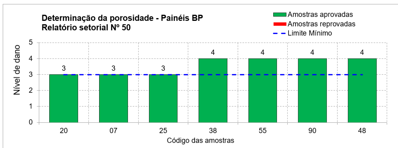
Figura 6 – Determinação da porosidade de painéis MDF com revestimento de 15 mm de espessura
