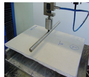
b. Ensaio de ruptura na flexão
