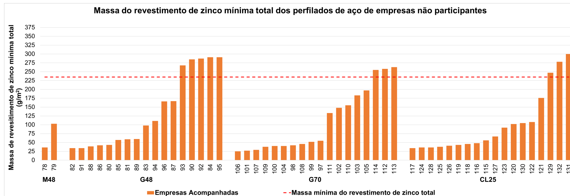
Figura 19 – Resultados da determinação da massa do revestimento de zinco total (nas duas faces) das amostras de perfilados de aço de empresas não participantes avaliadas
