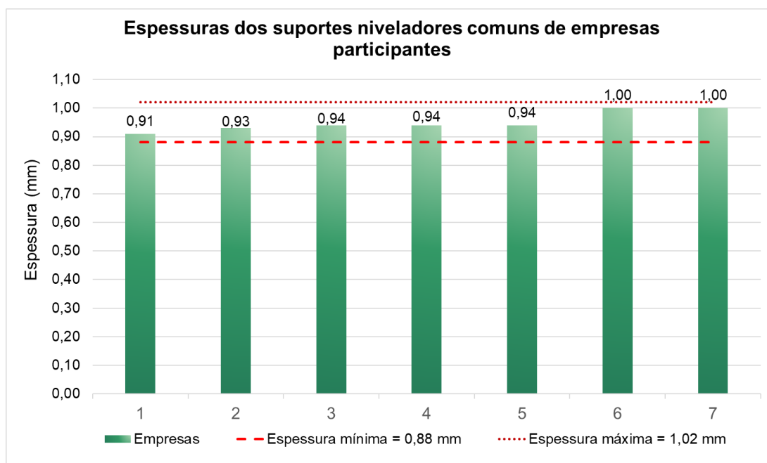
Figura 20 – Resultados da determinação da espessura das amostras de suporte nivelador comum avaliadas de empresas participantes
