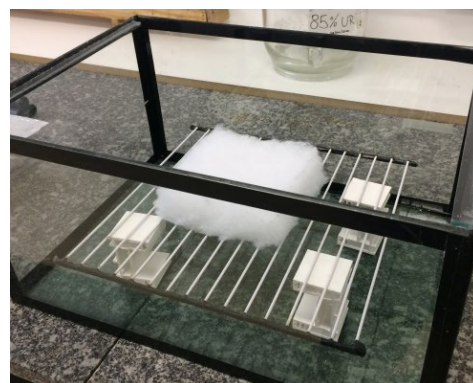
c. Ensaio de determinação da absorção de umidade
