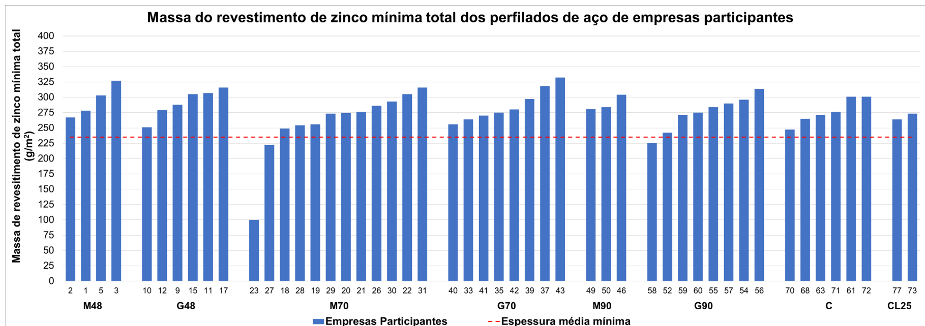
Figura 17 – Resultados da determinação da massa do revestimento de zinco total (nas duas faces) das amostras de perfilados de aço de empresas participantes avaliadas
