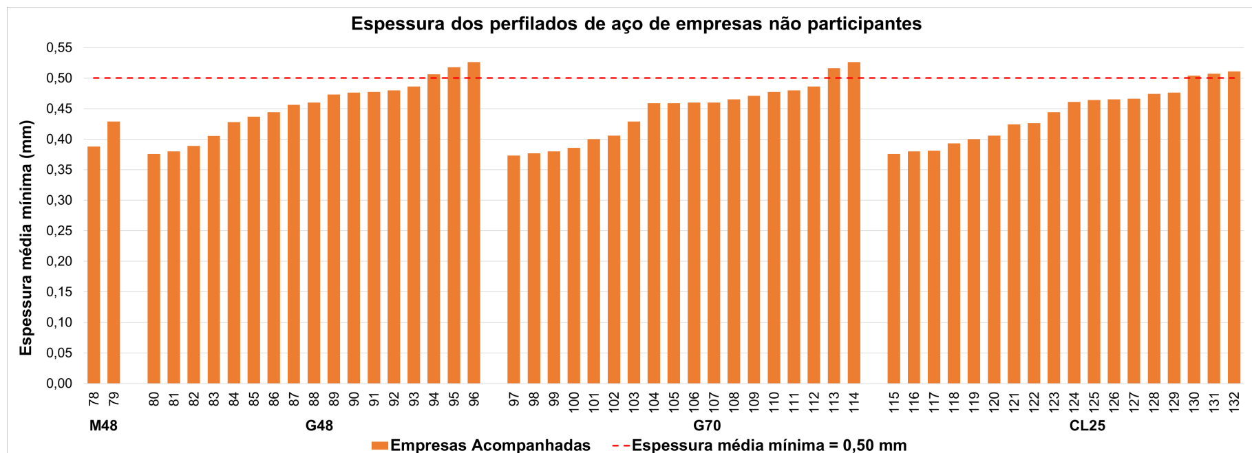
Figura 15 – Resultados da determinação da espessura das amostras de perfilados de aço de empresas não participantes avaliadas
