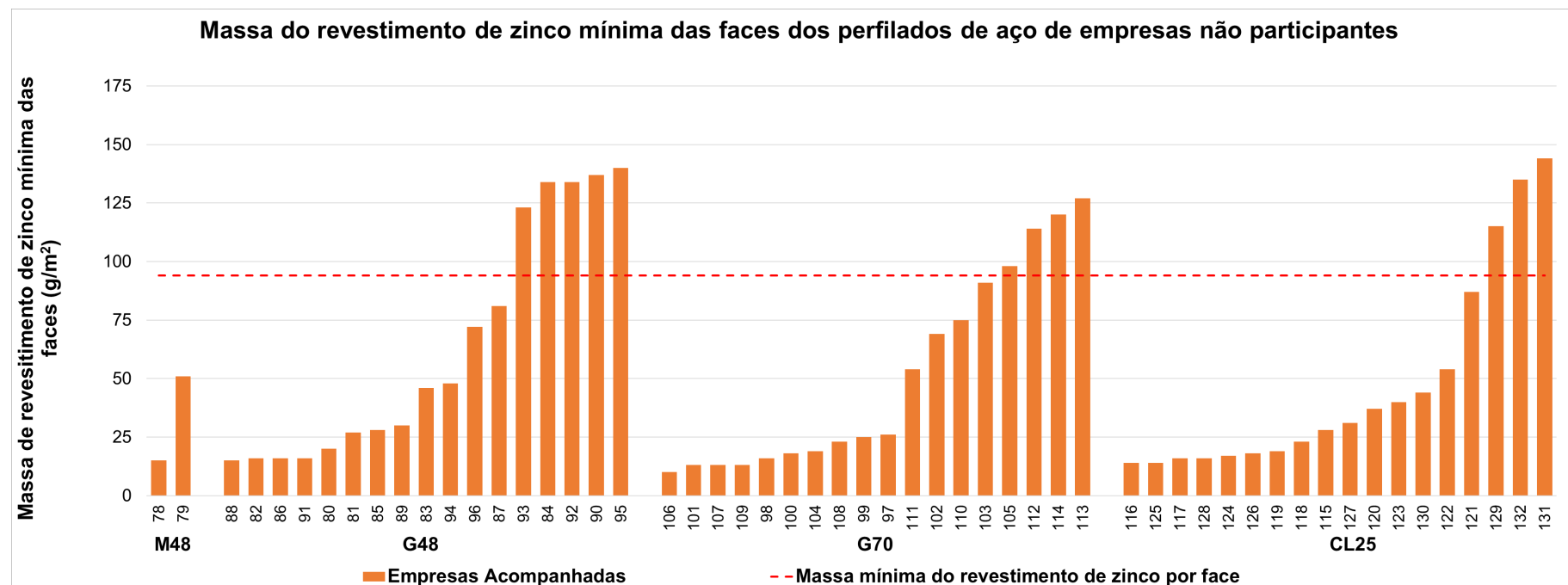
Figura 18 – Resultados da determinação da massa do revestimento de zinco mínima das faces das amostras de perfilados de aço de empresas não participantes avaliadas
