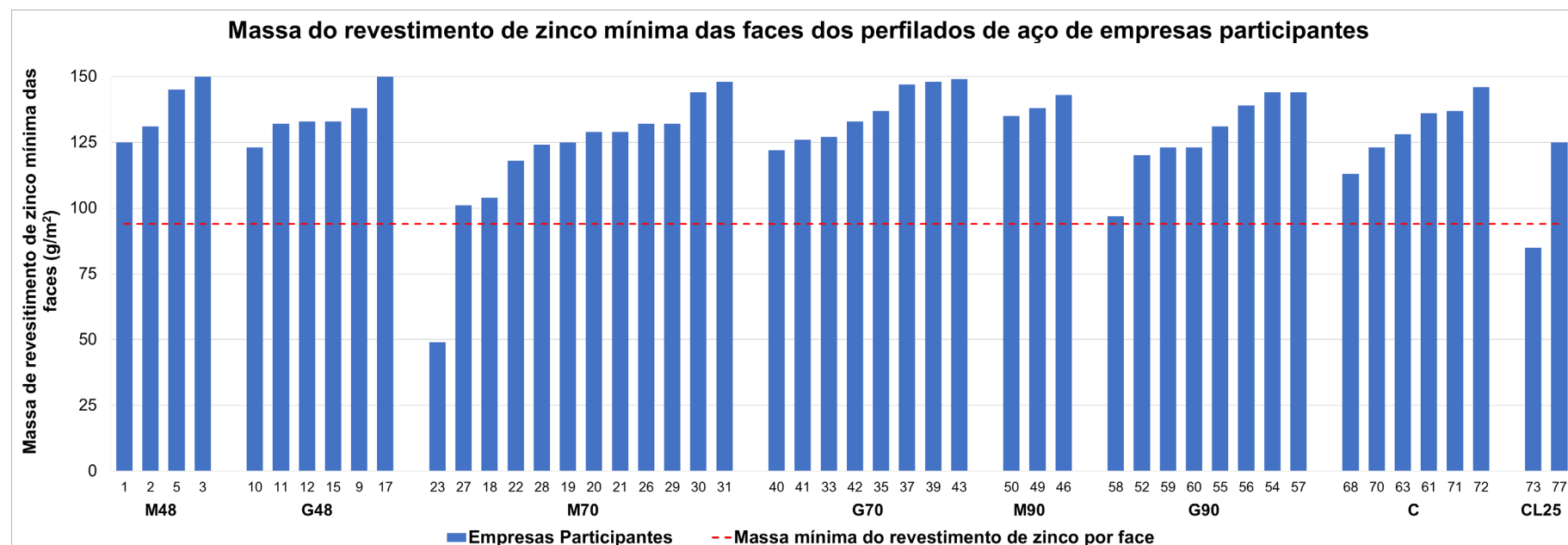
Figura 16 – Resultados da determinação da massa do revestimento de zinco mínima das faces das amostras de perfilados de aço de empresas participantes avaliadas
