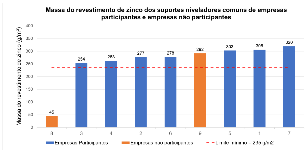
Figura 21 – Resultados da determinação da massa de revestimento de zinco das amostras de suporte nivelador comum avaliadas de empresas participantes e empresas não participantes (o resultado refere-se à média aritmética da massa de zinco de três suportes da mesma amostra)
