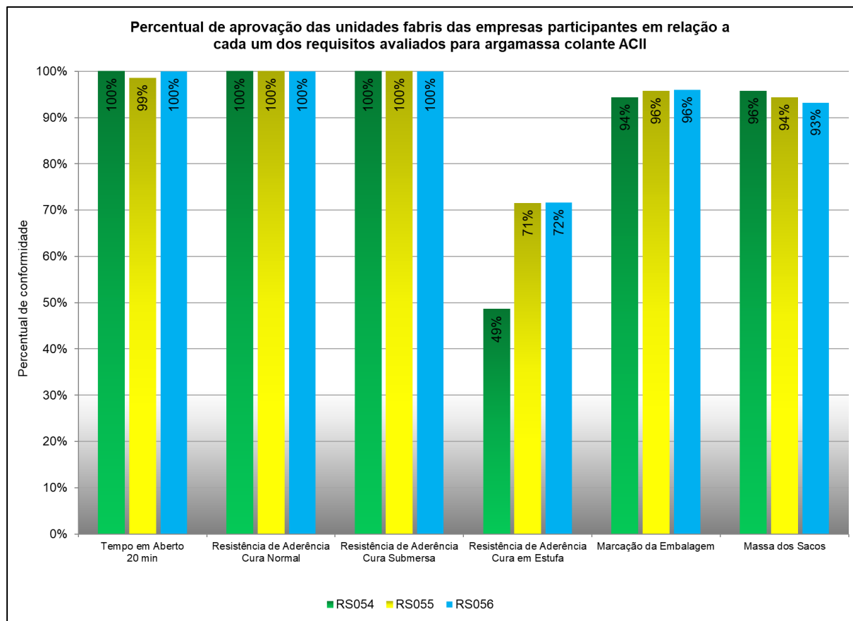
Figura 4 – Evolução das unidades fabris das empresas participantes do Programa para cada um dos requisitos avaliados para as argamassas colantes tipo ACII
