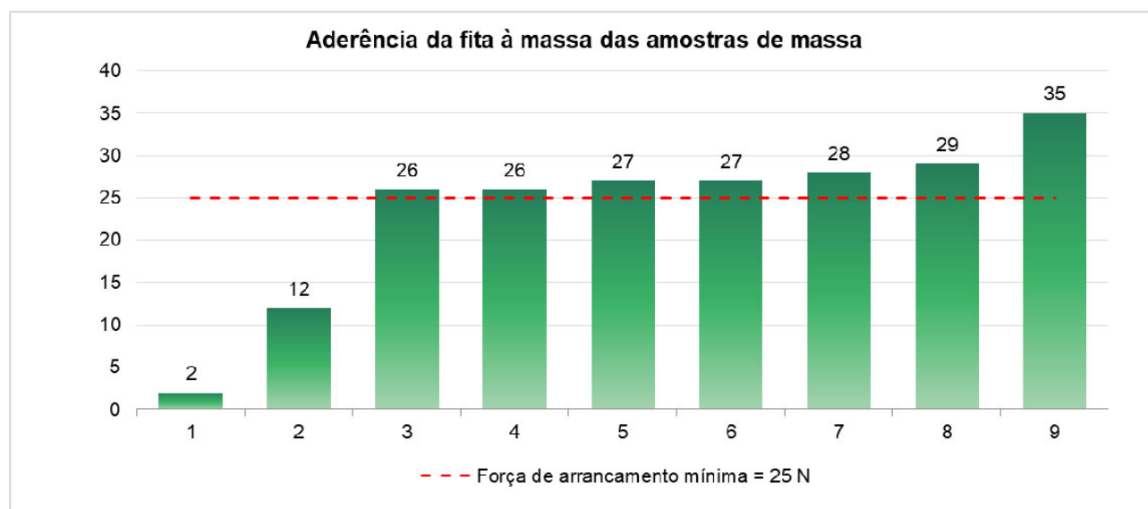
Figura 30 – Resultados da verificação da aderência da fita à massa das amostras de massa para tratamento de juntas avaliadas (empresas participantes e não participantes)
