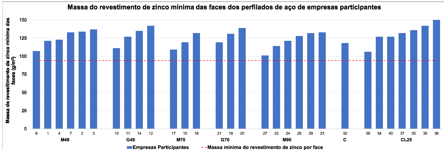
Figura 23 – Resultados da determinação da massa do revestimento de zinco mínima das faces das amostras de perfilados de aço de empresas participantes avaliadas
