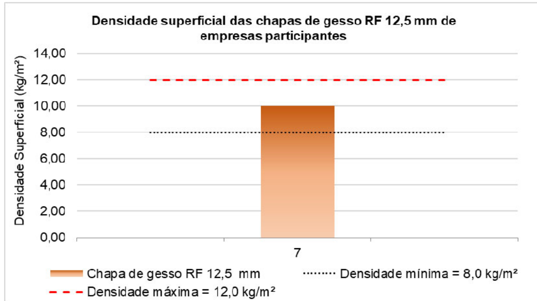
Figura 16 – Resultado da determinação da densidade superficial da amostra de chapa de gesso RF 12,5 mm avaliada
