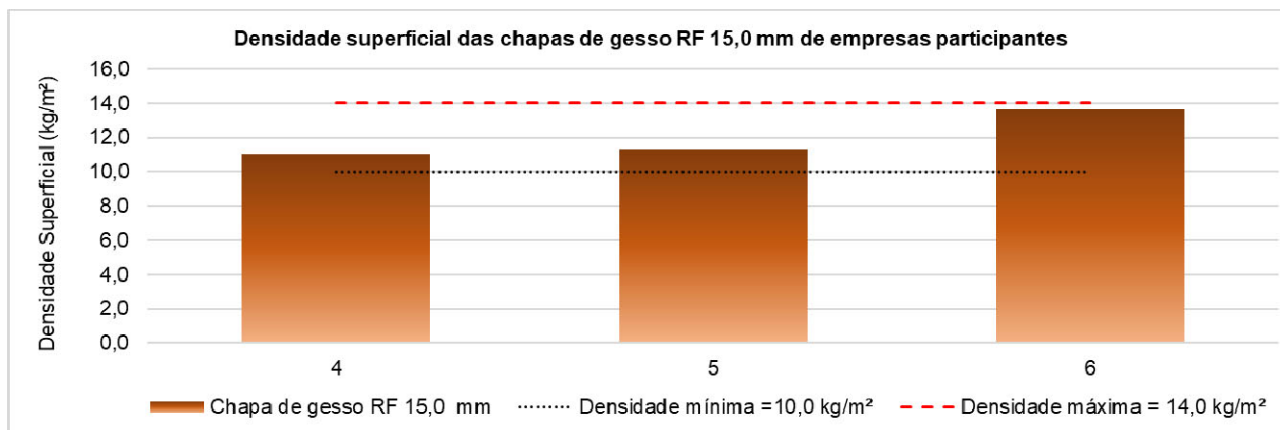
Figura 14 – Resultados da determinação da densidade superficial das amostras de chapas de gesso RF 15,0 mm avaliadas
