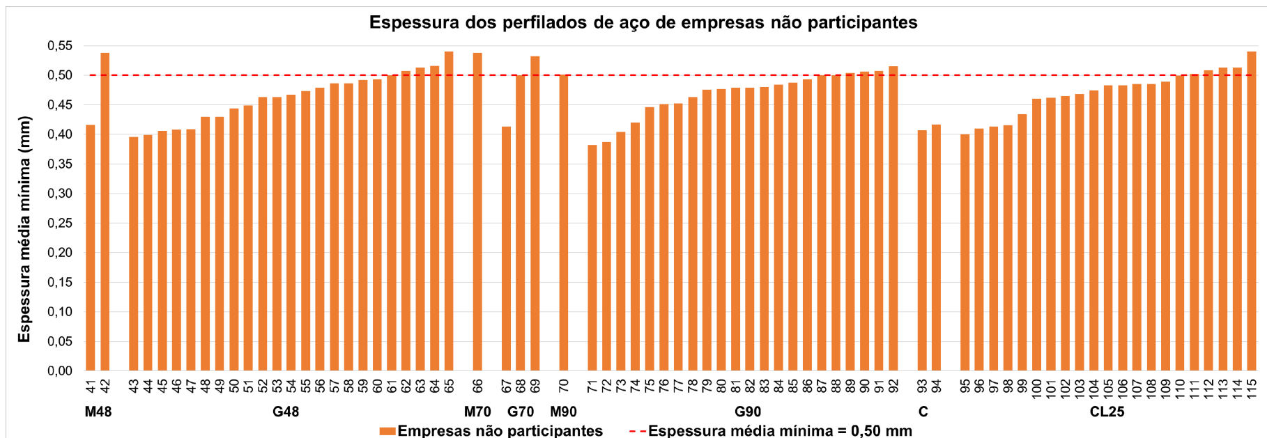
Figura 22 – Resultados da determinação da espessura das amostras de perfilados de aço de empresas não participantes avaliadas
