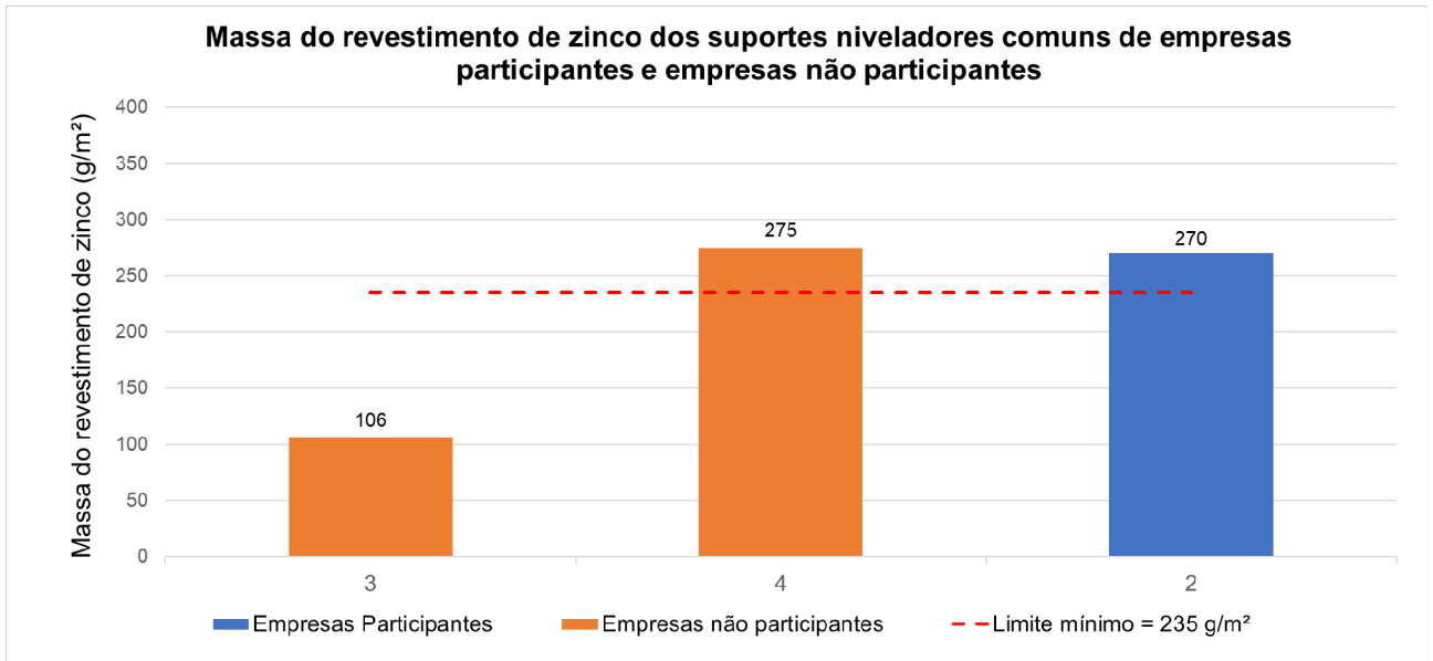
Figura 28 – Resultados da determinação da massa de revestimento de zinco das amostras de suporte nivelador comum avaliadas de empresas participantes e empresas não participantes (o resultado refere-se à média aritmética da massa de zinco de três suportes da mesma amostra)
