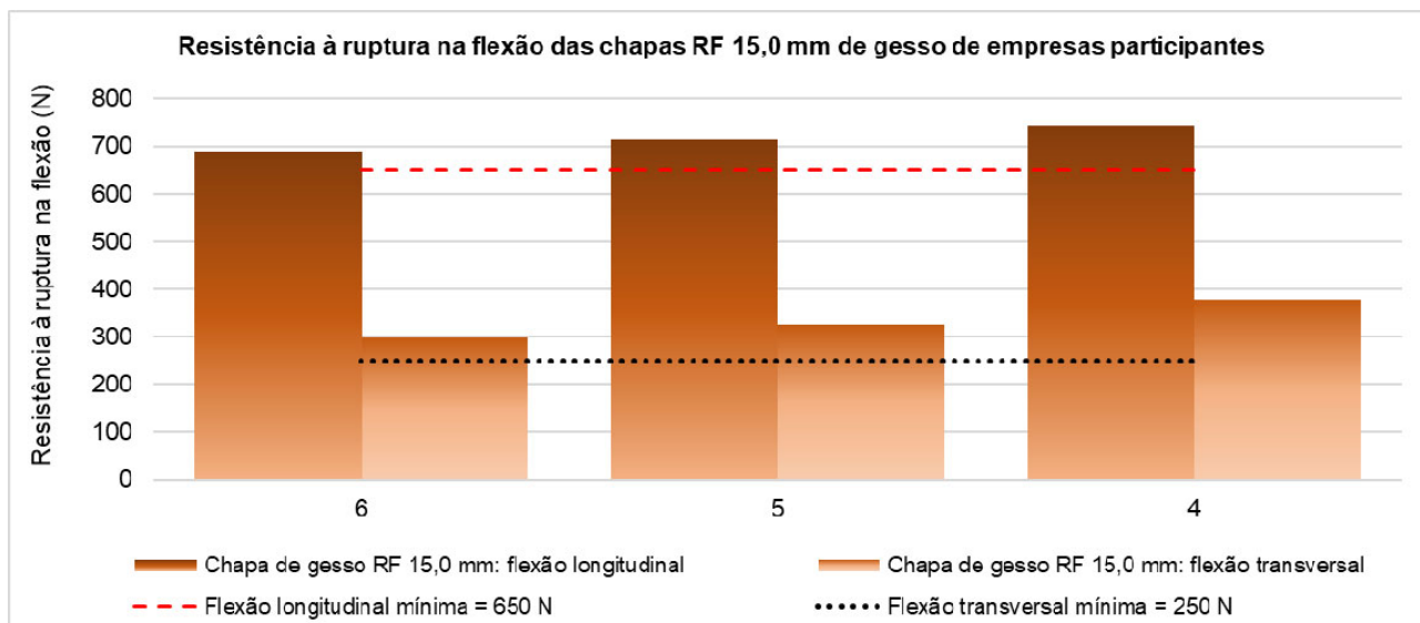
Figura 15 – Resultados da determinação da resistência à flexão (média) das amostras de chapas de gesso RF 15,0 mm avaliadas
