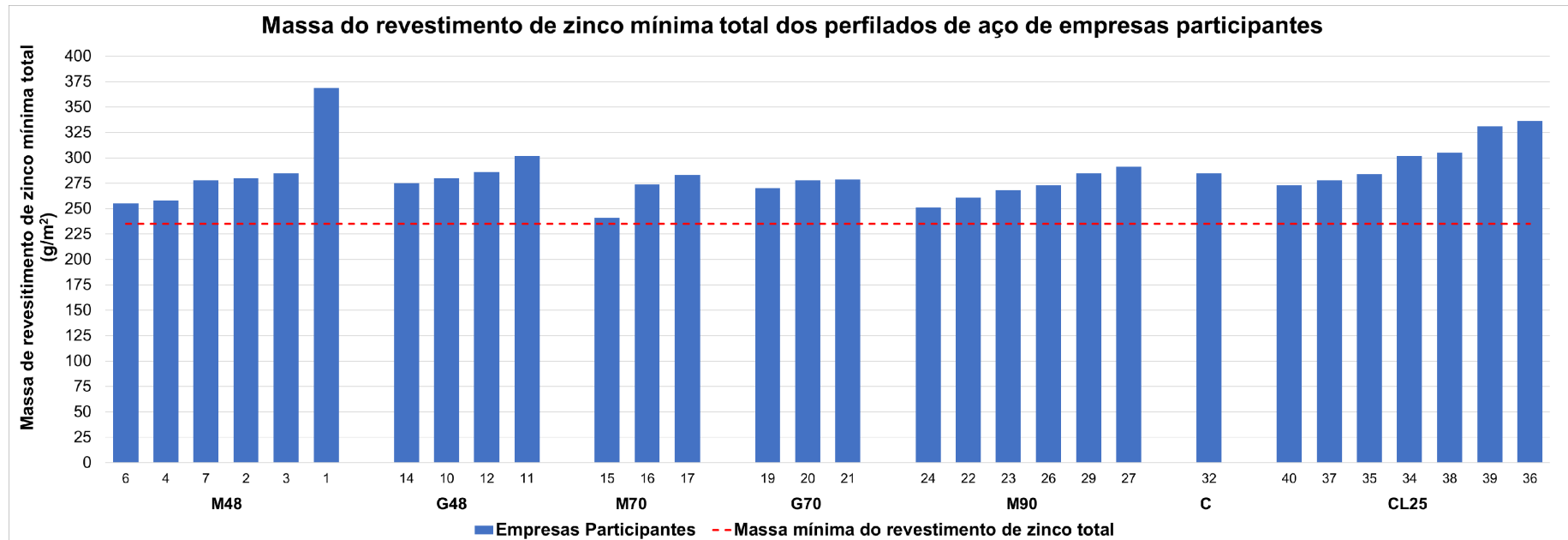
Figura 24 – Resultados da determinação da massa do revestimento de zinco total (nas duas faces) das amostras de perfilados de aço de empresas participantes avaliadas
