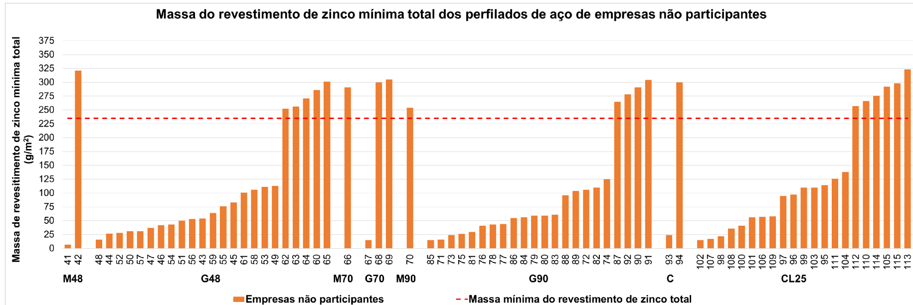
Figura 26 – Resultados da determinação da massa do revestimento de zinco total (nas duas faces) das amostras de perfilados de aço de empresas não participantes avaliadas
