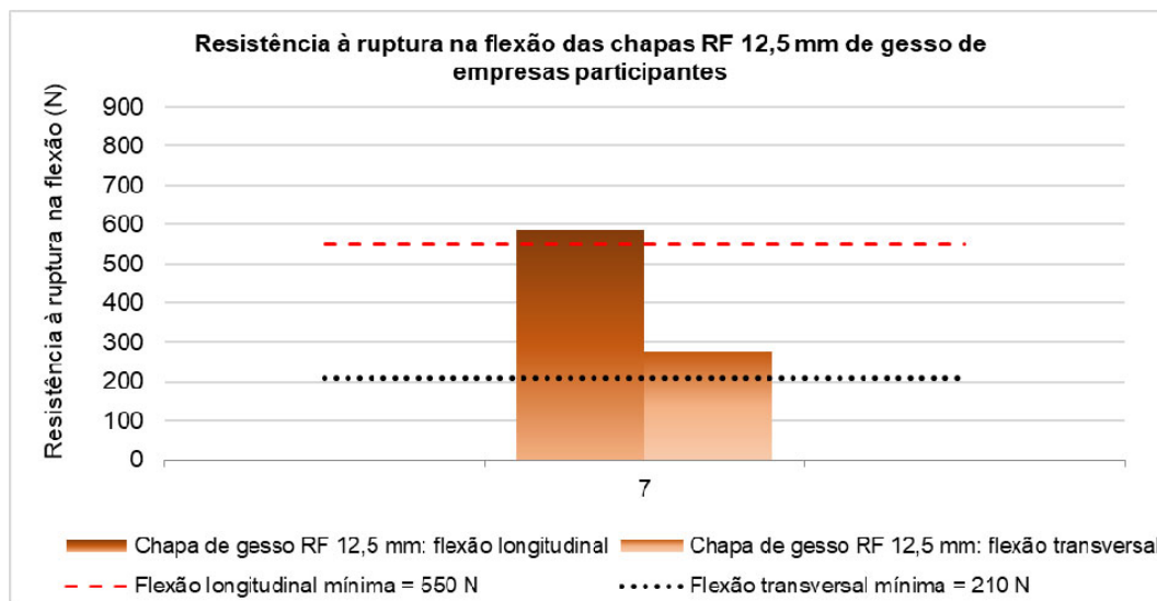
Figura 177 – Resultados da determinação da resistência à flexão (média) da amostra de chapa de gesso RF 12,5 mm avaliada
