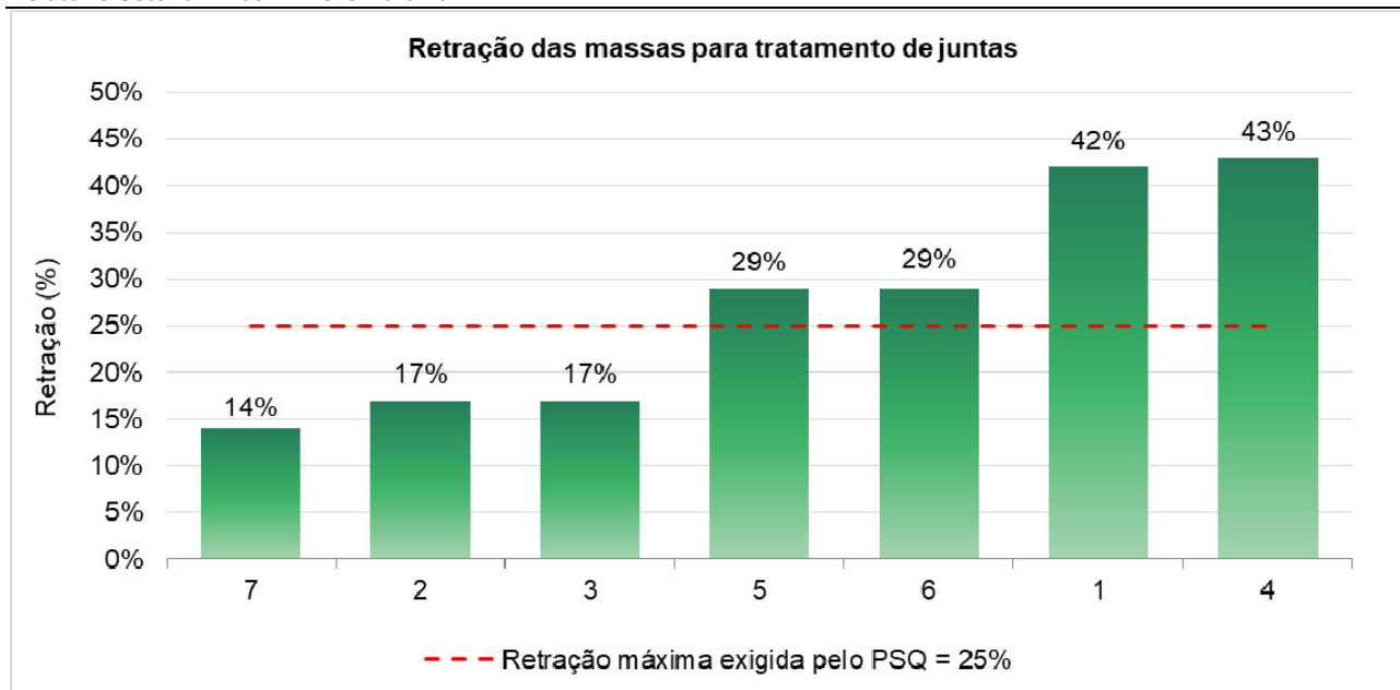
Figura 31 – Resultados da verificação da retração das amostras de massa para tratamento de juntas avaliadas (empresas participantes e não participantes)
