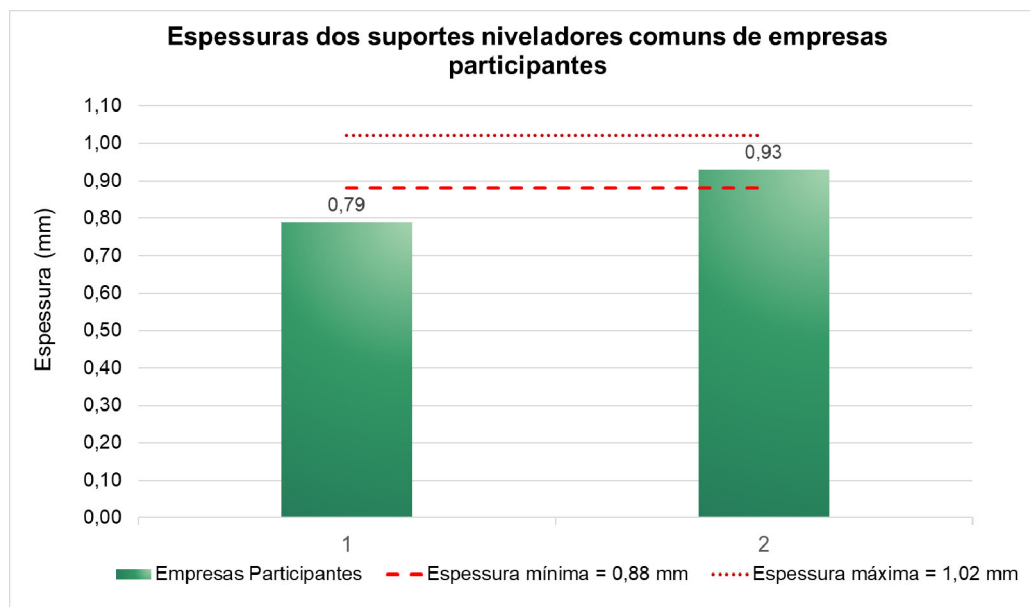
Figura 27 – Resultados da determinação da espessura das amostras de suporte nivelador comum avaliadas de empresas participantes
