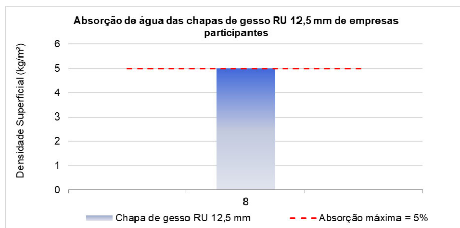
Figura 20 – Resultados da absorção de água de chapas de gesso RU 12,5 mm avaliadas
