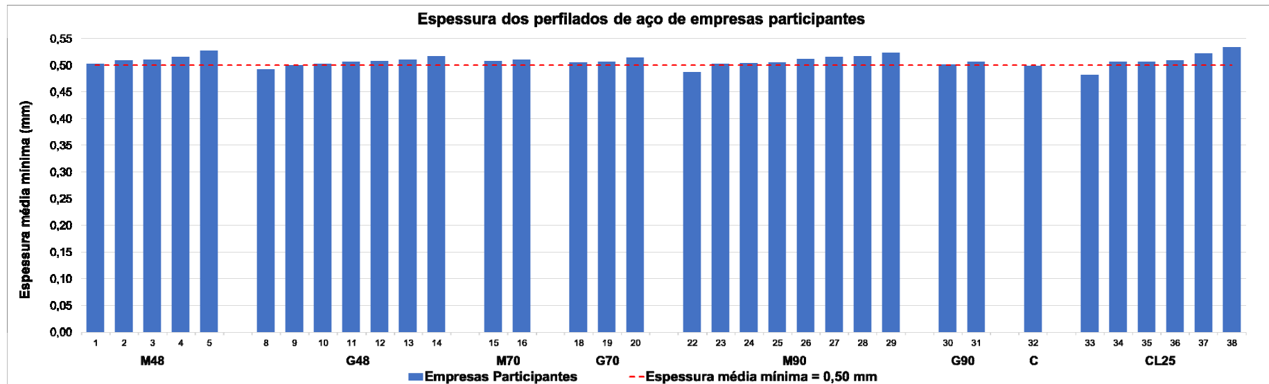
Figura 21 – Resultados da determinação da espessura das amostras de perfilados de aço de empresas participantes avaliadas
