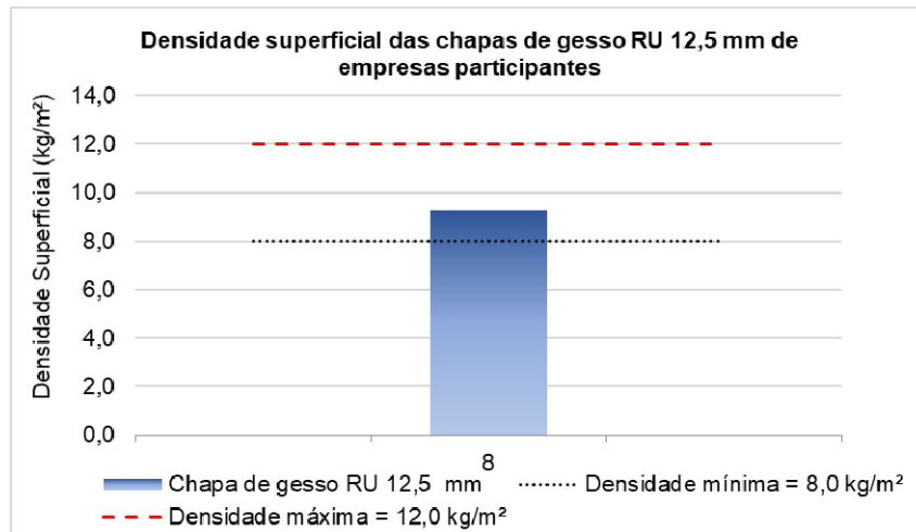
Figura 188 – Resultado da determinação da densidade superficial da amostra de chapa de gesso RU 12,5 mm avaliada
