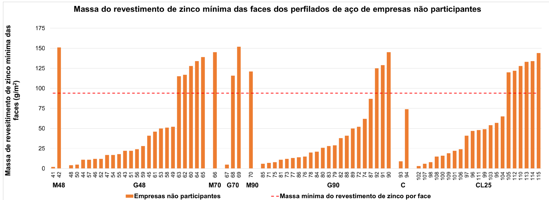
Figura 25 – Resultados da determinação da massa do revestimento de zinco mínima das faces das amostras de perfilados de aço de empresas não participantes avaliadas
