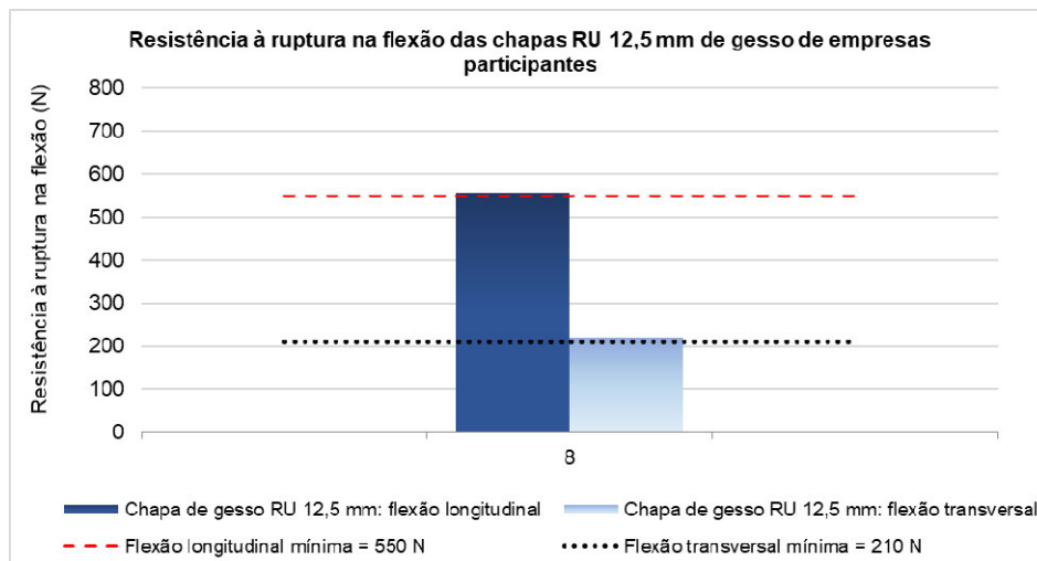
Figura 199 – Resultados da determinação da resistência à flexão (média) da amostra de chapa de gesso RU 12,5 mm avaliada
