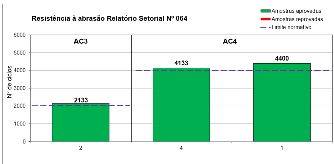
Figura 5 - Resultados obtidos no ensaio de determinação da resistência à abrasão em pisos laminados melamínicos de classe de abrasão AC3 e AC4 produzidos por empresas participantes
