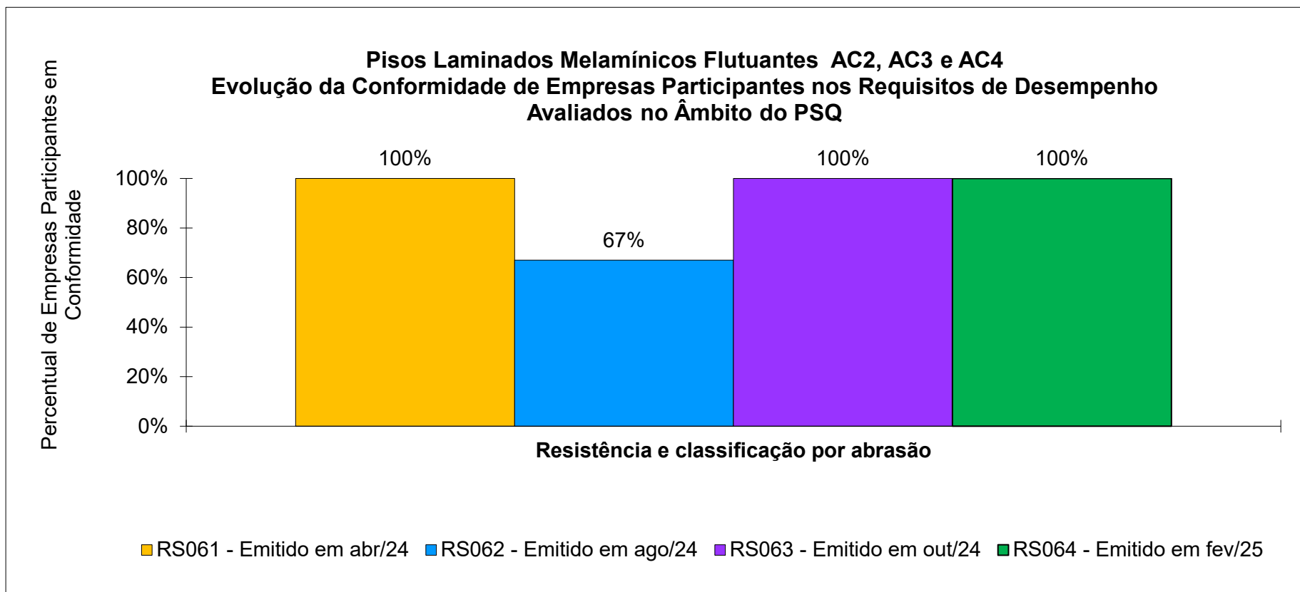
Figura 11 - Evolução da qualidade dos pisos laminados melamínicos flutuantes de classes de abrasão AC2, AC3 e AC4 de empresas PARTICIPANTES, para cada análise realizada no âmbito do Programa Setorial da Qualidade
