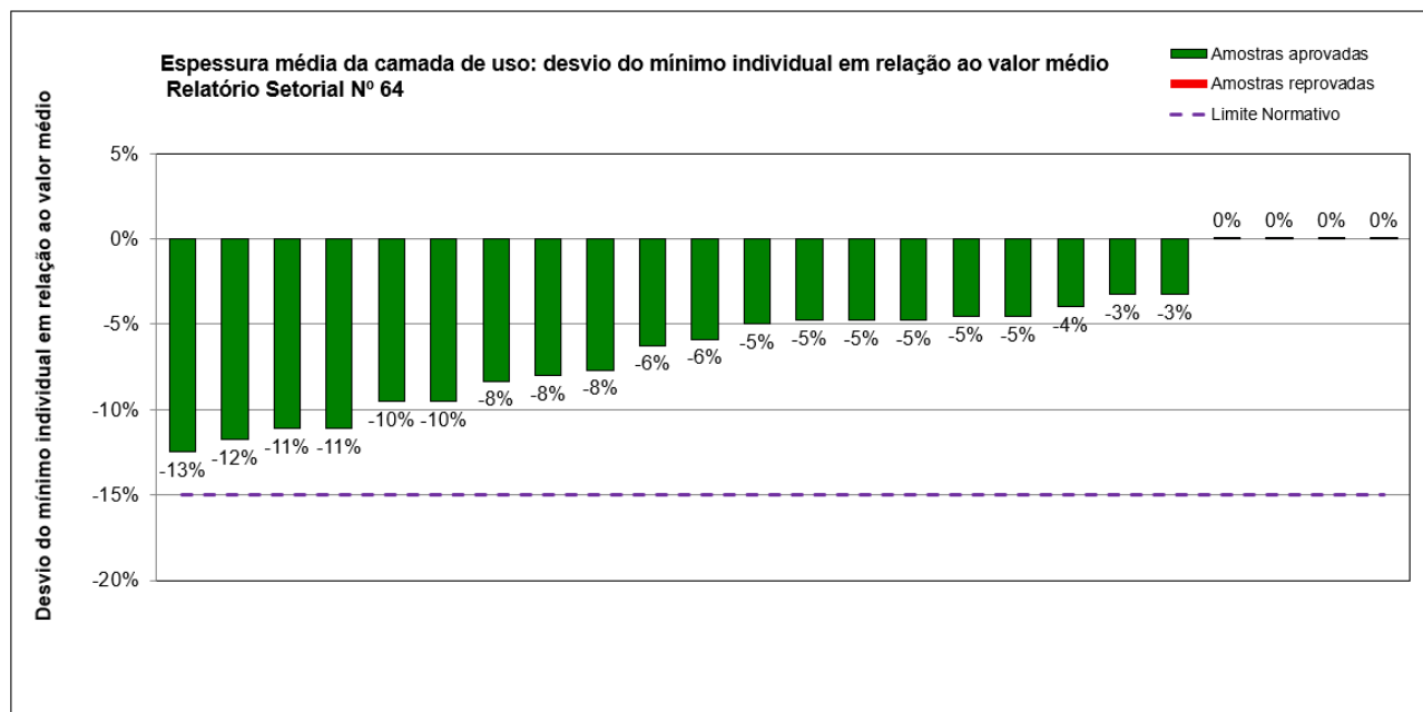
Figura 8 - Resultados obtidos no ensaio de determinação da espessura nominal média da camada de uso em pisos laminados vinílicos produzidos por empresas participantes e não participantes
