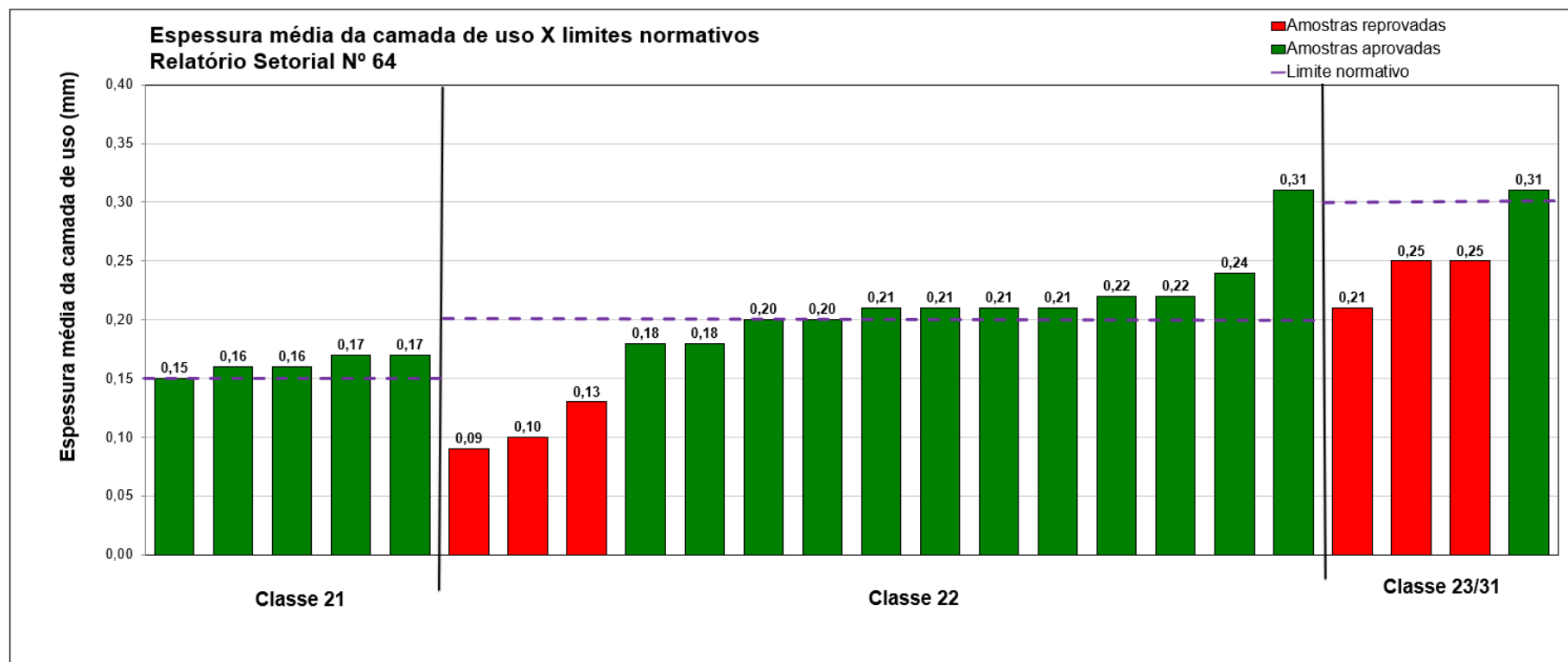
Figura 6 - Resultados obtidos no ensaio de determinação da espessura nominal média da camada de uso em pisos laminados vinílicos produzidos por empresas participantes e não participantes
