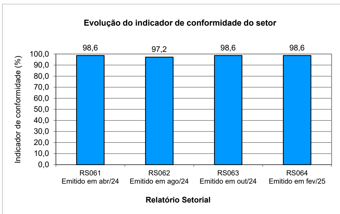
Figura 13 - Evolução do indicador de conformidade do setor de pisos laminados fornecidos em régua, considerando exclusivamente pisos laminados melamínicos flutuantes de classes de abrasão AC2, AC3 e AC4
