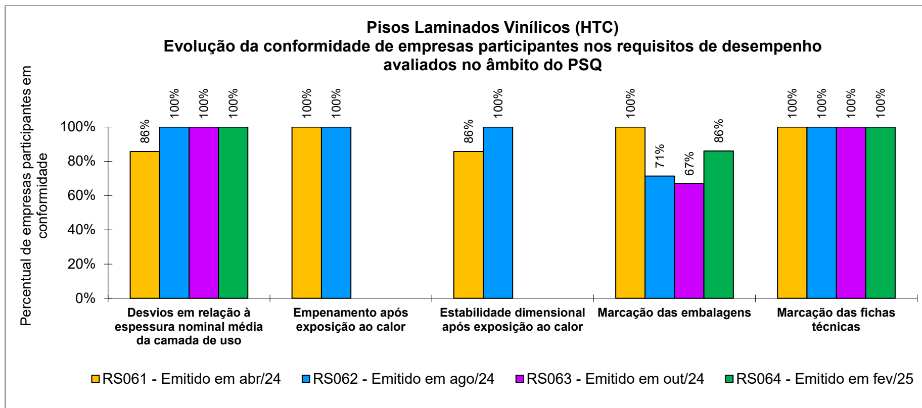
Figura 12 - Evolução da qualidade dos pisos laminados vinílicos heterogêneos de base compacta (HTC) de empresas PARTICIPANTES, para cada análise realizada no âmbito do Programa Setorial da Qualidade
