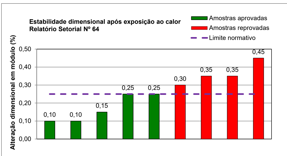
Figura 10 - Resultados obtidos no ensaio de determinação da estabilidade dimensional após exposição ao calor em pisos laminados vinílicos produzidos por empresas participantes e não participantes
