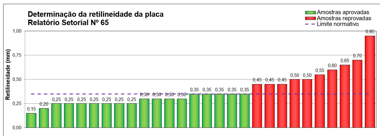
Figura 12 - Resultados obtidos no ensaio de determinação da retilidade em pisos laminados vinílicos produzidos por empresas participantes e não participantes
