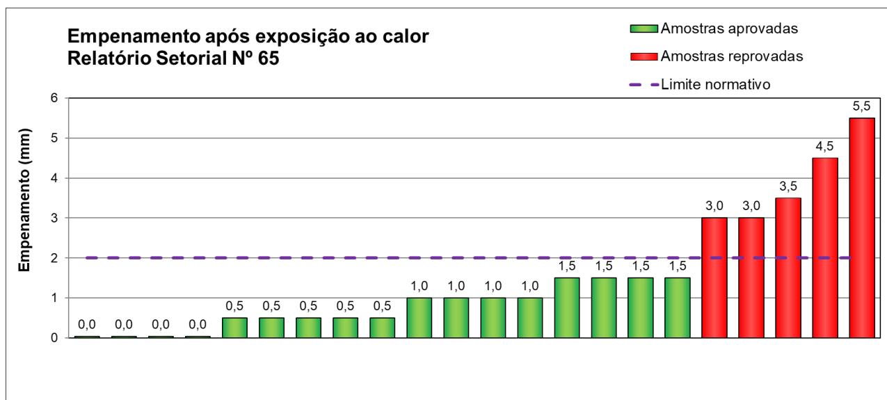
Figura 9 - Resultados obtidos no ensaio de determinação do empenamento após exposição ao calor em pisos laminados vinílicos produzidos por empresas participantes e não participantes
