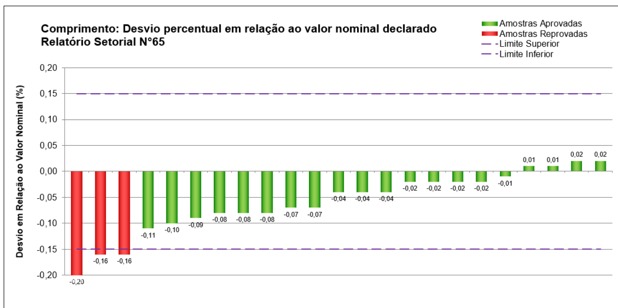
Figura 14 - Resultados obtidos no ensaio de determinação do comprimento em pisos laminados vinílicos produzidos por empresas participantes e não participantes (desvio em relação ao valor nominal – %)
