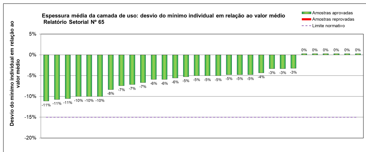
Figura 8 - Resultados obtidos no ensaio de determinação da espessura nominal média da camada de uso em pisos laminados vinílicos produzidos por empresas participantes e não participantes
