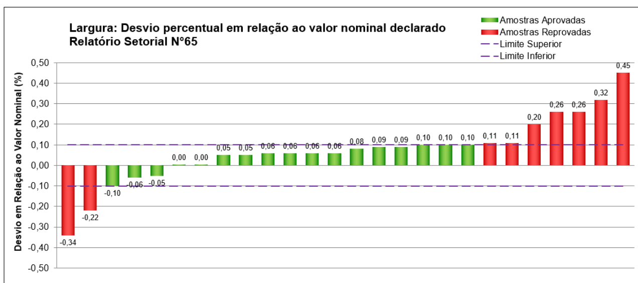
Figura 16 - Resultados obtidos no ensaio de determinação da largura em pisos laminados vinílicos produzidos por empresas participantes e não participantes (desvio em relação ao valor nominal – %)
