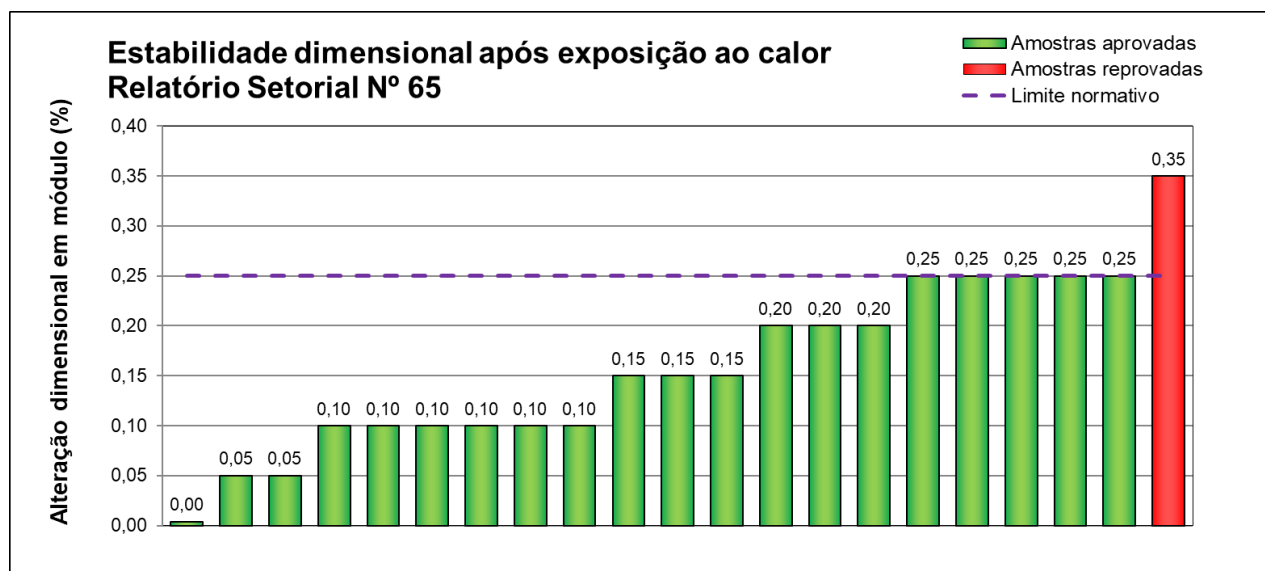
Figura 10 - Resultados obtidos no ensaio de determinação da estabilidade dimensional após exposição ao calor em pisos laminados vinílicos produzidos por empresas participantes e não participantes
