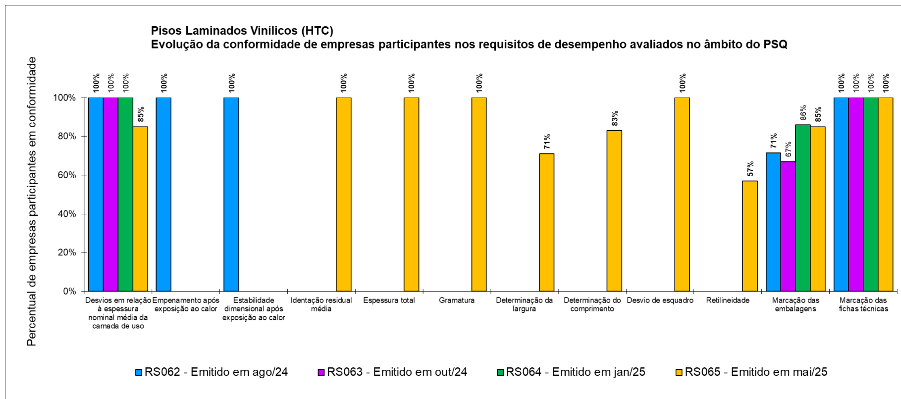
Figura 22 - Evolução da qualidade dos pisos laminados vinílicos heterogêneos de base compacta (HTC) de empresas PARTICIPANTES, para cada análise realizada no âmbito do Programa Setorial da Qualidade
