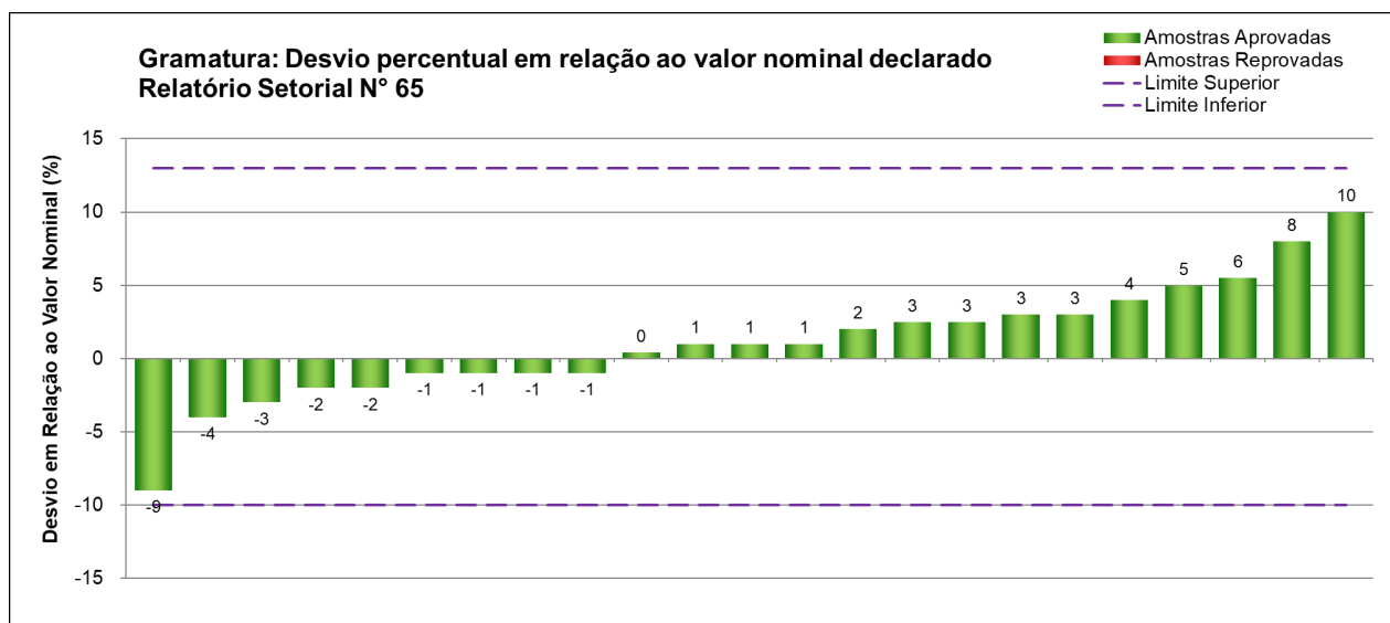
Figura 19 - Resultados obtidos no ensaio de determinação da massa por unidade de área (gramatura) em pisos laminados vinílicos produzidos por empresas participantes e não participantes
