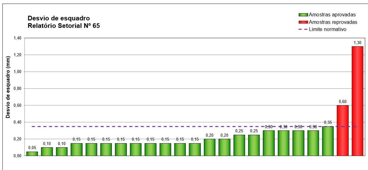
Figura 11 - Resultados obtidos no ensaio de determinação do desvio de esquadro em pisos laminados vinílicos produzidos por empresas participantes e não participantes
