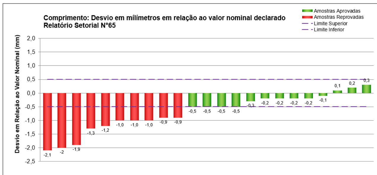
Figura 13 - Resultados obtidos no ensaio de determinação do comprimento em pisos laminados vinílicos produzidos por empresas participantes e não participantes (desvio em relação ao valor nominal – mm)
