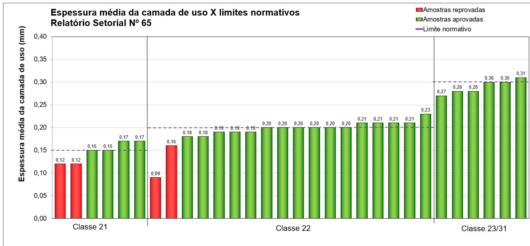
Figura 6 - Resultados obtidos no ensaio de determinação da espessura nominal média da camada de uso em pisos laminados vinílicos produzidos por empresas participantes e não participantes
