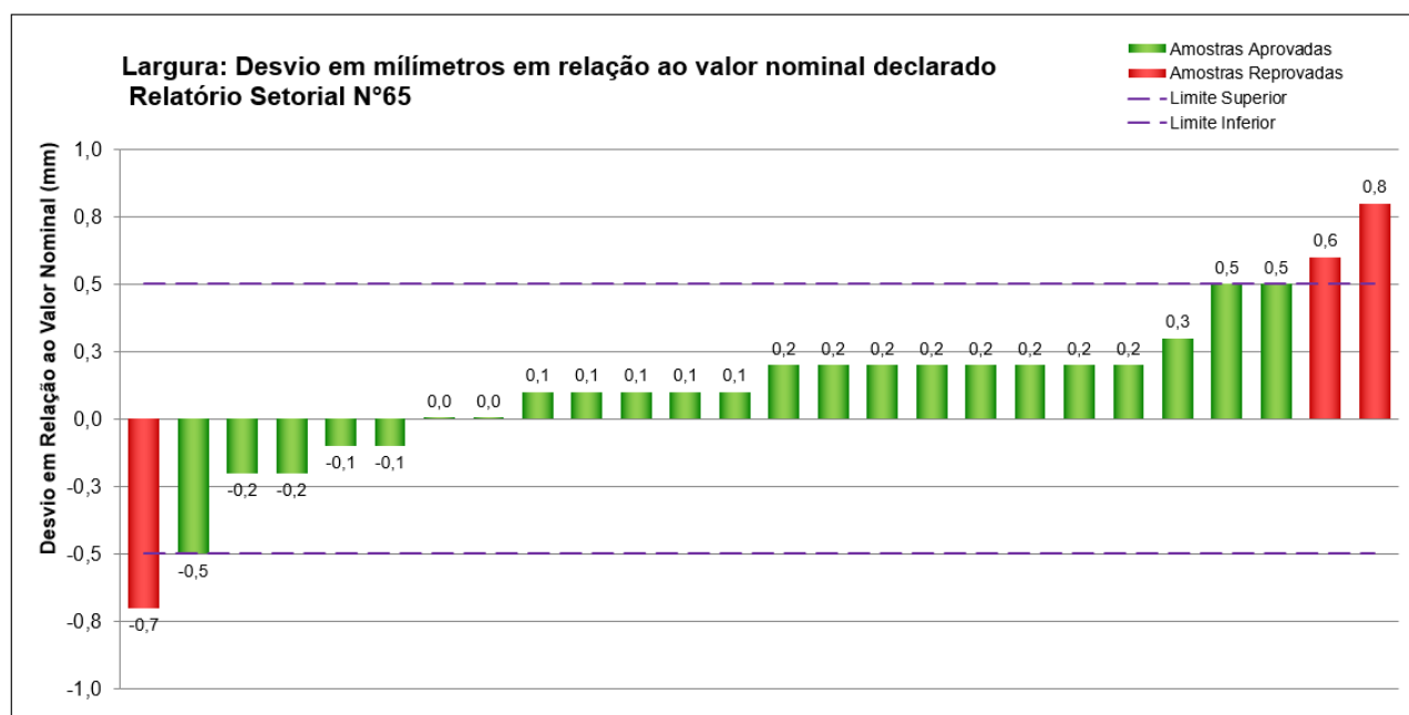
Figura 15 - Resultados obtidos no ensaio de determinação da largura em pisos laminados vinílicos produzidos por empresas participantes e não participantes (desvio em relação ao valor nominal – mm)
