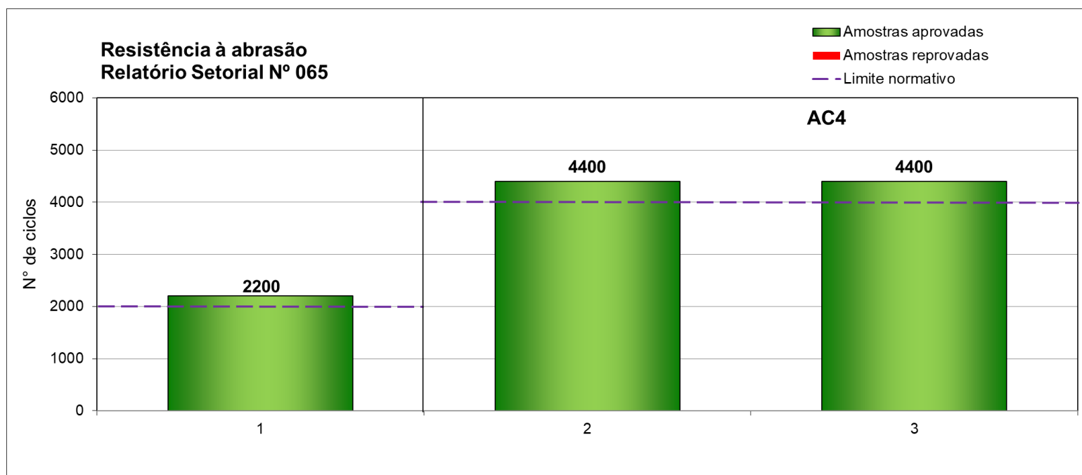
Figura 5 - Resultados obtidos no ensaio de determinação da resistência à abrasão em pisos laminados melamínicos de classe de abrasão AC3 e AC4 produzidos por empresas participantes
