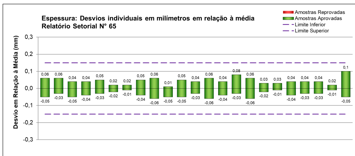
Figura 18 - Resultados obtidos no ensaio de determinação da espessura total em pisos laminados vinílicos produzidos por empresas participantes e não participantes (desvios individuais em relação à média)
