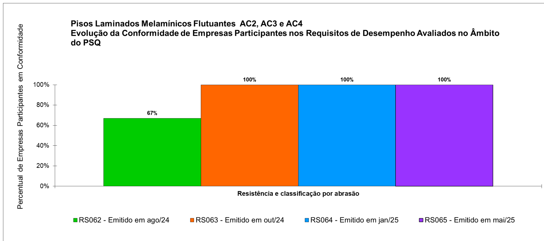
Figura 21 - Evolução da qualidade dos pisos laminados melamínicos flutuantes de classes de abrasão AC2, AC3 e AC4 de empresas PARTICIPANTES, para cada análise realizada no âmbito do Programa Setorial da Qualidade
