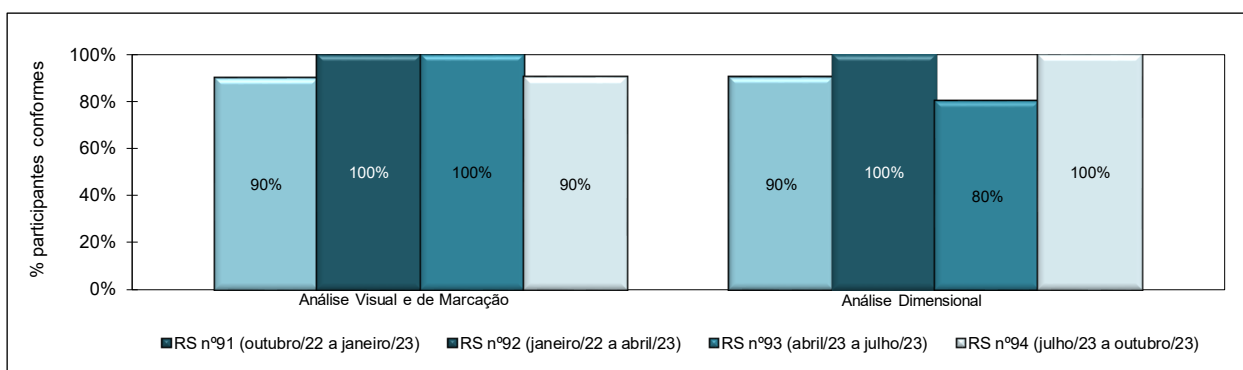
Figura 2 – Evolução da conformidade das bacias sanitárias das empresas participantes - Análises visual e dimensional
