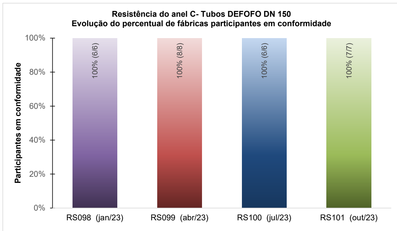
Figura 6 – Resistência do anel C dos tubos DEFOFO DN 150
