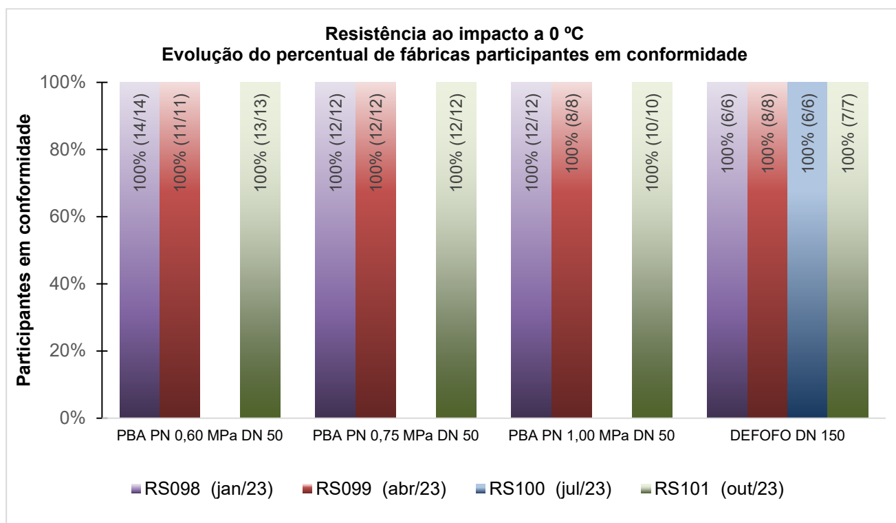
Figura 4 – Resistência ao impacto de tubos de PVC para infraestrutura
