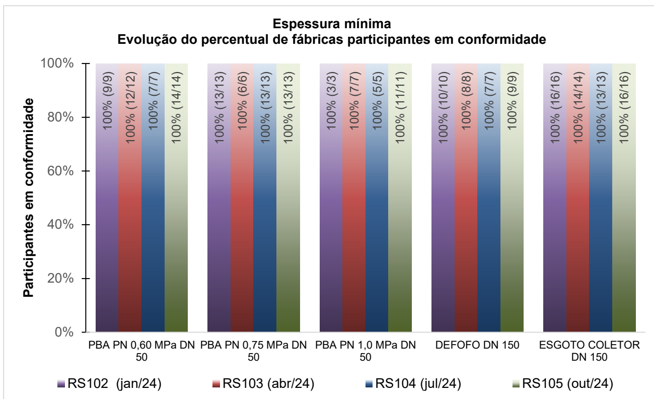
Figura 2 – Espessura mínima de lotes de tubos de PVC para infraestrutura
