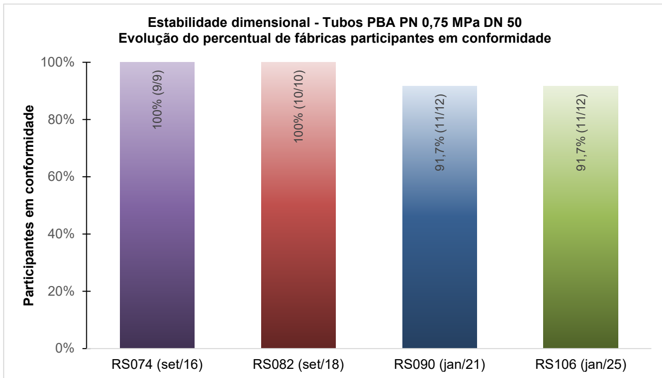
Figura 7 – Verificação da estabilidade dimensional dos tubos PBA PN 0,75 MPa DN 50
