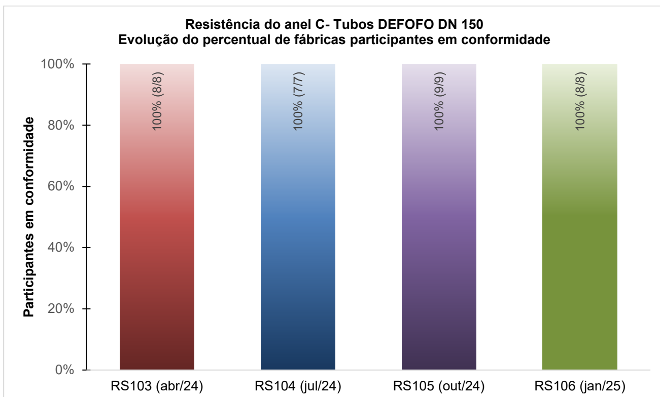
Figura 6 – Resistência do anel C dos tubos DEFOFO DN 150
