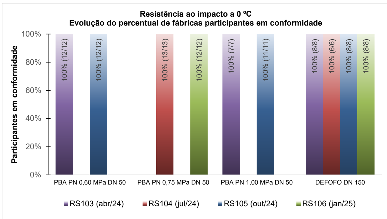
Figura 4 – Resistência ao impacto a 0° de tubos de PVC para infraestrutura
