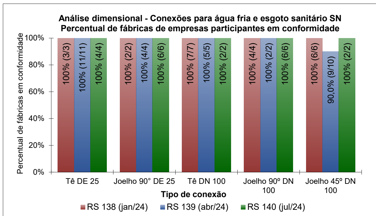
Figura 11 - Análise dimensional de conexões para água fria e esgoto sanitário SN
