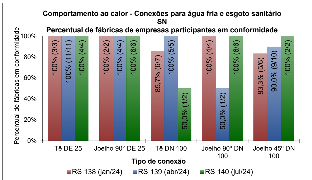
Figura 12 - Verificação do comportamento ao calor das conexões para água fria e esgoto sanitário SN
