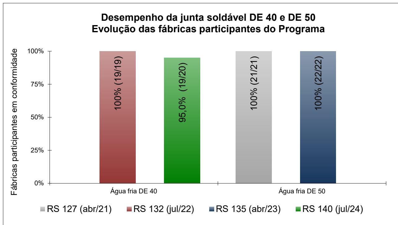
Figura 9 - Verificação da junta soldável dos tubos para água fria DE 40
