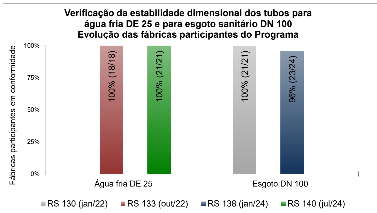
Figura 8 - Verificação da estabilidade dimensional dos tubos para água fria DE 25
