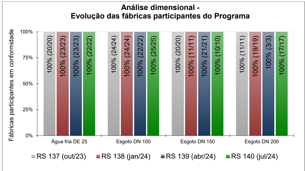
Figura 2 - Análise dimensional dos tubos para água fria DE 25 e tubos para esgoto sanitário SN DN 100, DN 150 e DN 200
