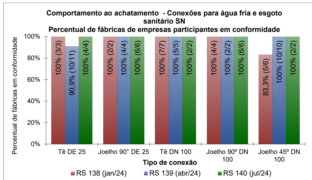
Figura 13 - Verificação do comportamento ao achatamento das conexões para água fria e esgoto sanitário SN
