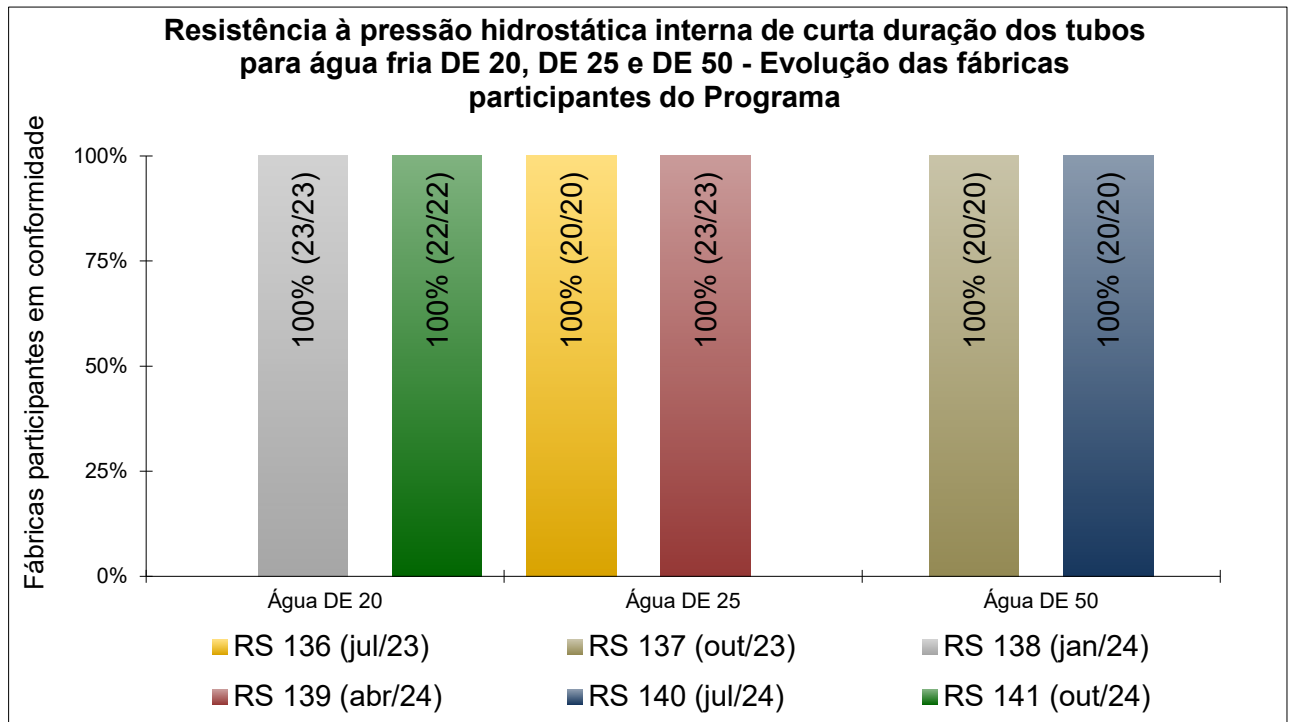
Figura 4 - Verificação da resistência à pressão hidrostática interna de curta duração dos tubos para água fria DE 20, DE 25 e DE 50
