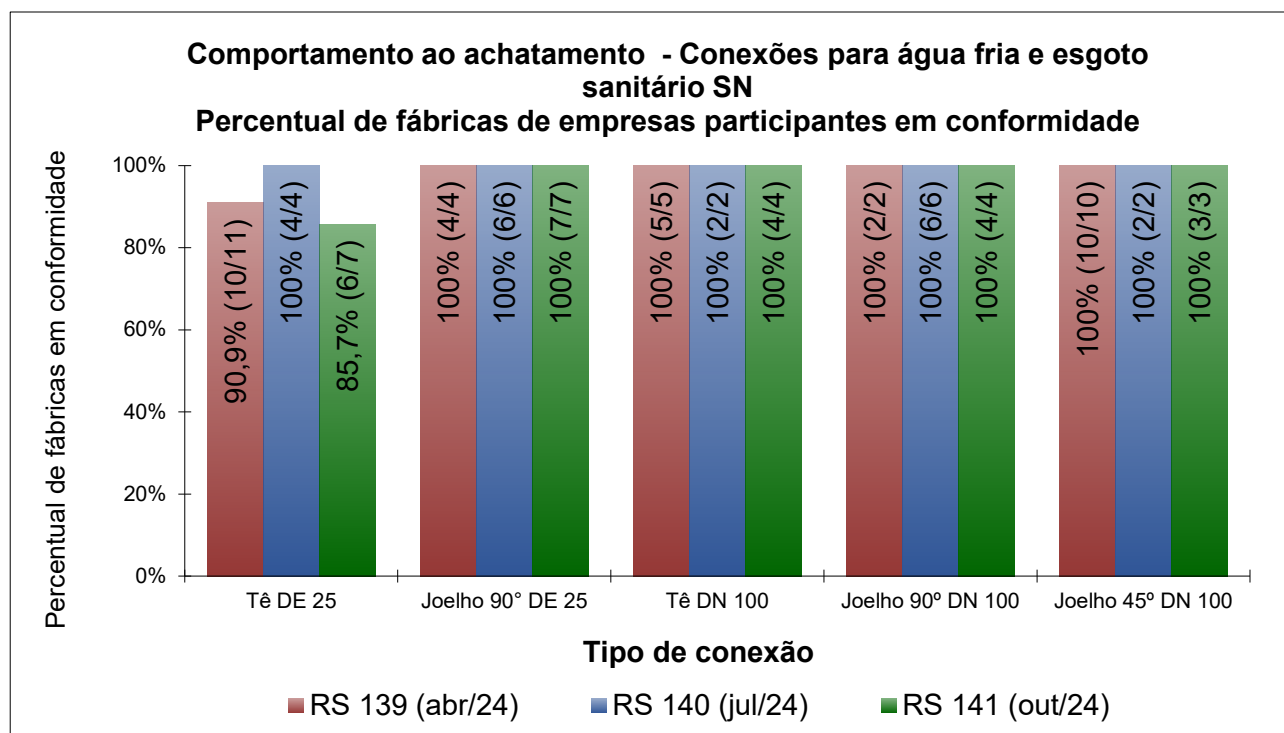
Figura 11 - Verificação do comportamento ao achatamento das conexões para água fria e esgoto sanitário SN
