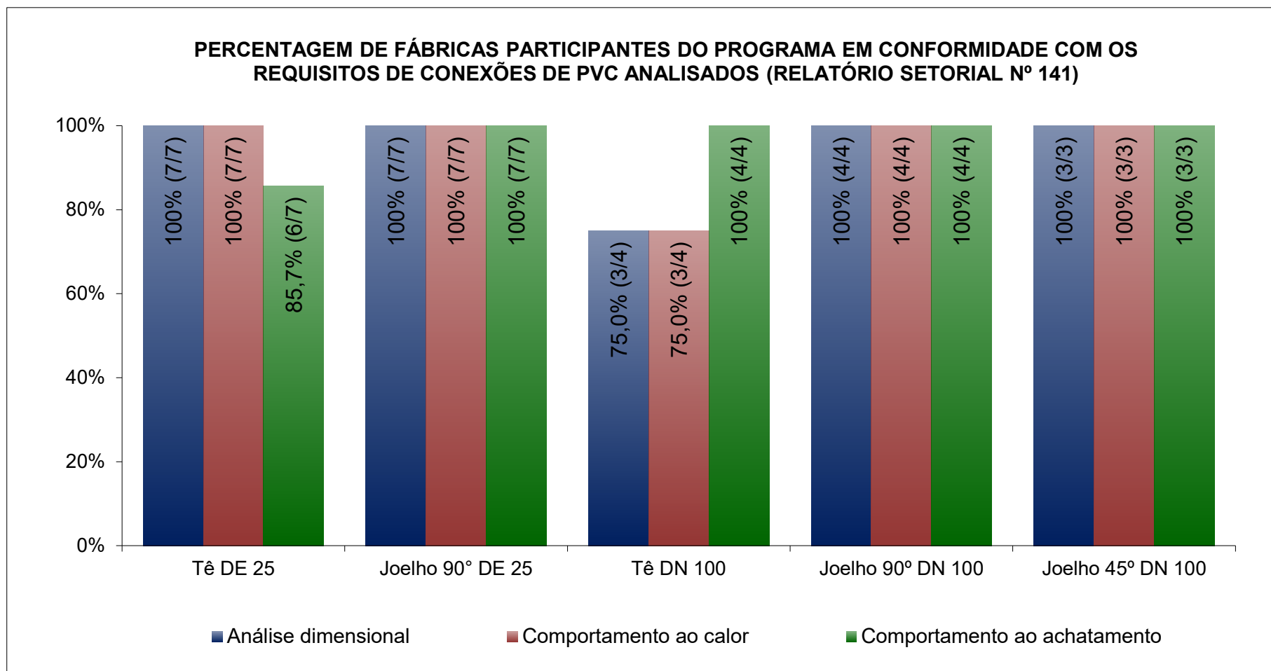
Figura 12 - Conexões de PVC - Fábricas participantes em conformidade com os requisitos analisados pelo Programa Setorial da Qualidade – Relatório Setorial nº 141
