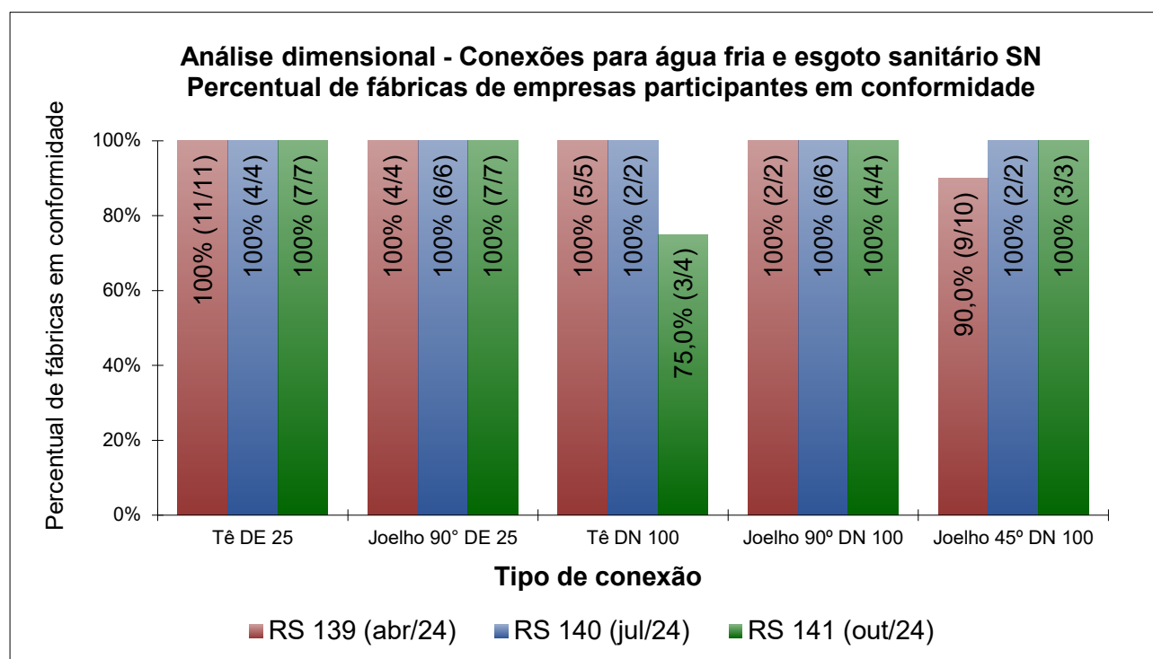
Figura 9 - Análise dimensional de conexões para água fria e esgoto sanitário SN
