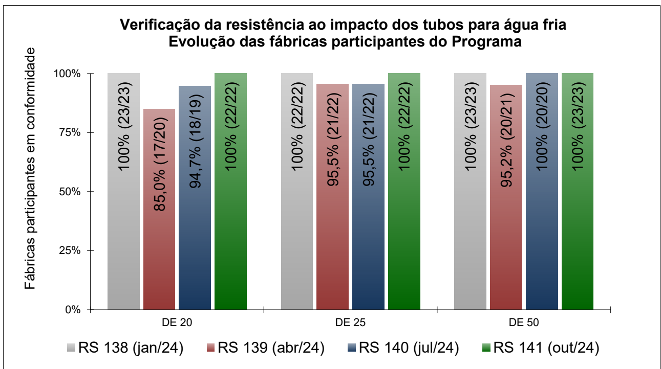
Figura 5 - Verificação da resistência ao impacto a 0°C dos tubos para água fria DE 20, DE 25 e DE 50
