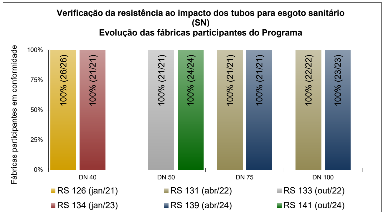
Figura 6 - Verificação da resistência ao impacto a 0°C dos tubos para esgoto sanitário SN DN 40, DN 50, DN 75 e DN 100
