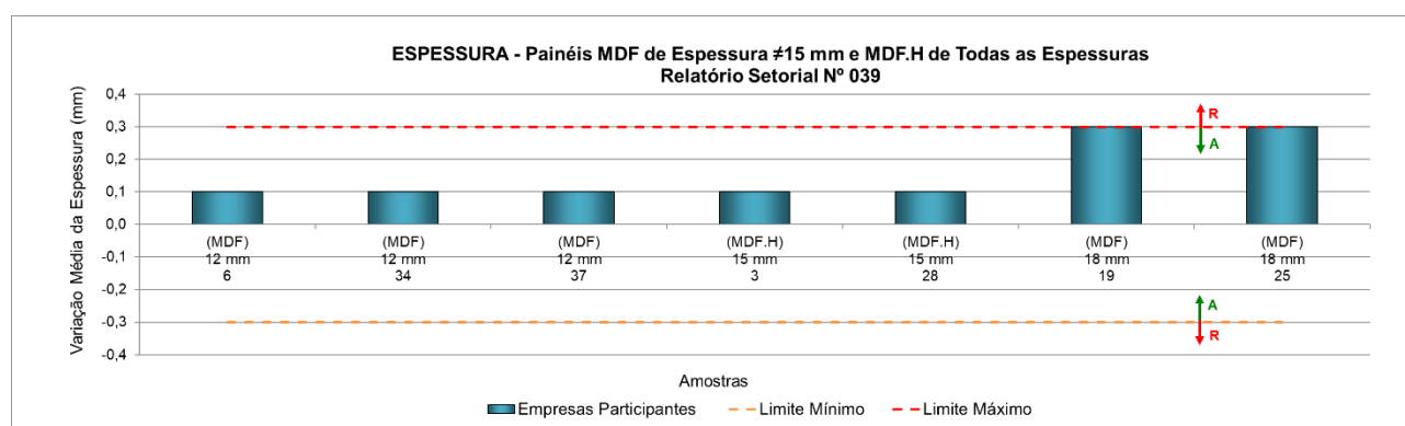
Figura 5 – Variação média da espessura de painéis MDF sem revestimento de espessuras diferentes de 15 mm e painéis MDF.H de todas as espessuras
