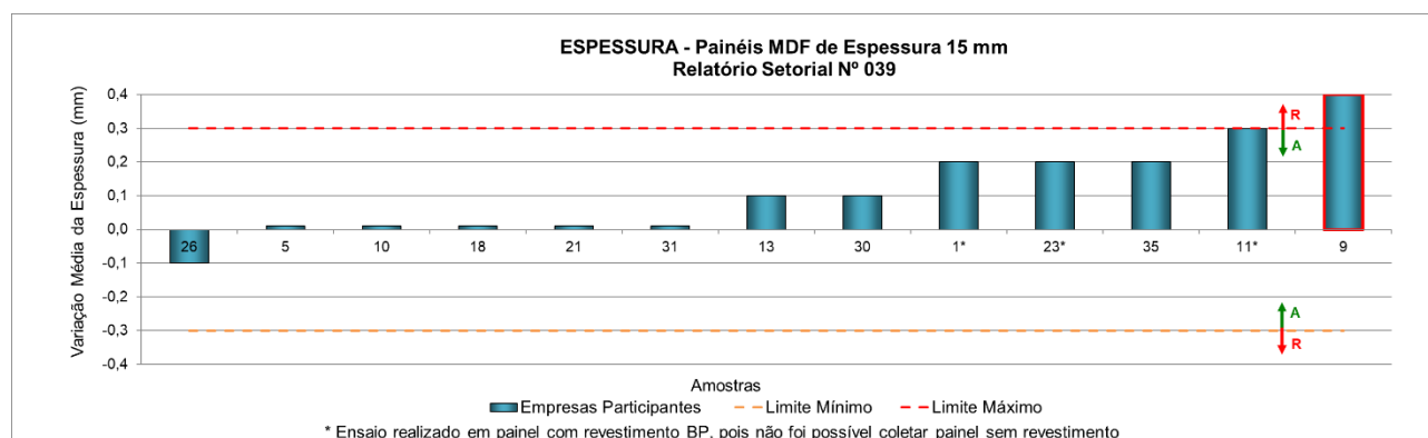
Figura 4 – Variação média da espessura de painéis MDF sem revestimento de 15 mm de espessura
