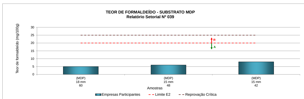
Figura 27 – Teor de formaldeído (método perforator ) de chapas de MDP utilizadas na fabricação de painéis revestidos
