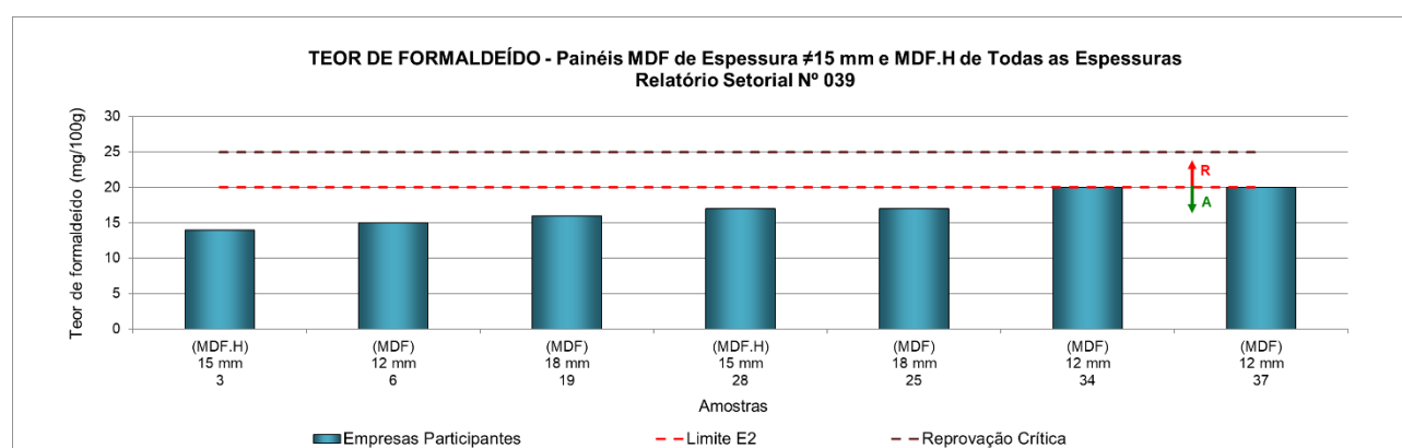
Figura 3 – Teor de formaldeído (método perforator ) de painéis MDF sem revestimento de espessuras diferentes de 15 mm e painéis MDF.H de todas as espessuras
