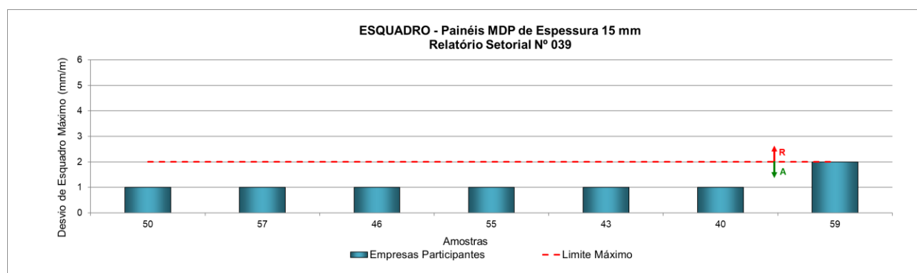
Figura 21 – Desvio de esquadro de painéis MDP sem revestimento de 15 mm de espessura
