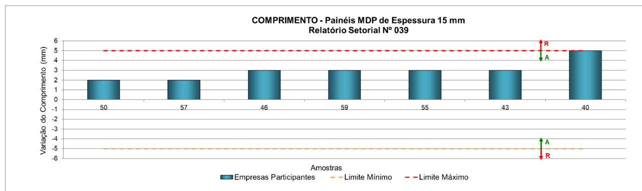
Figura 20 – Variação do comprimento de painéis MDP sem revestimento de 15 mm de espessura
