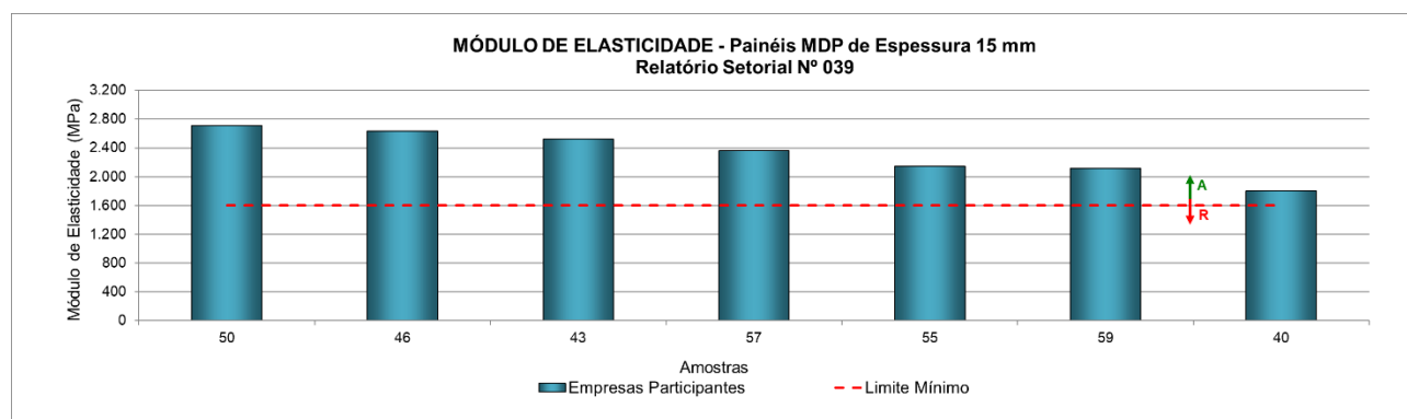
Figura 24 – Módulo de elasticidade de painéis MDP sem revestimento de 15 mm de espessura
