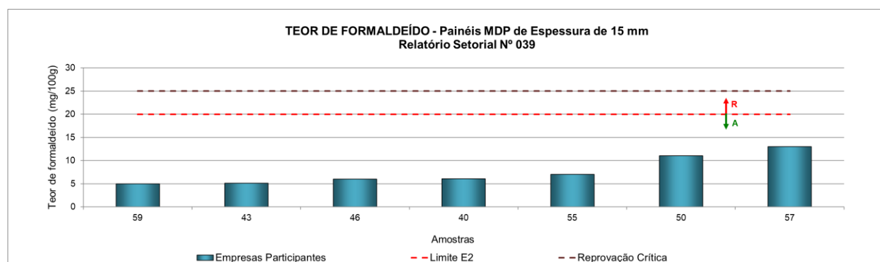
Figura 15 – Teor de formaldeído (método perforator ) de painéis MDP sem revestimento de 15 mm de espessura
