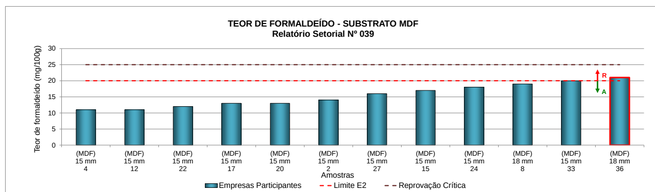
Figura 14 – Teor de formaldeído (método perforator ) de chapas de MDF utilizadas na fabricação de painéis revestidos
