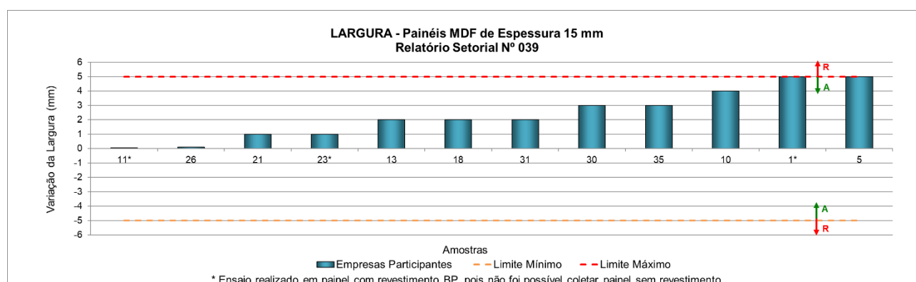
Figura 6 – Variação da largura de painéis MDF sem revestimento de 15 mm de espessura
