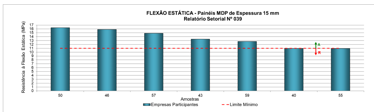
Figura 23 – Resistência à flexão estática de painéis MDP sem revestimento de 15 mm de espessura
