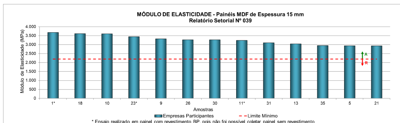
Figura 11 – Módulo de elasticidade de painéis MDF sem revestimento de 15 mm de espessura
