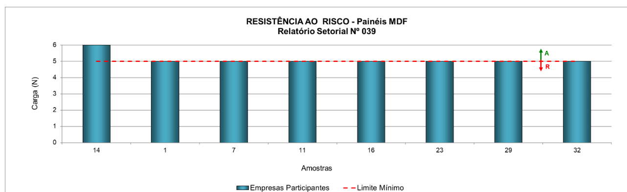
Figura 12 – Resistência ao risco de painéis MDF com revestimento BP, nas duas faces, de 15 mm de espessura
