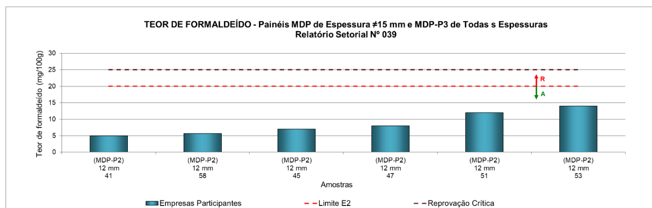
Figura 16 – Teor de formaldeído (método perforator ) de painéis MDP sem revestimento de espessuras diferentes de 15 mm
