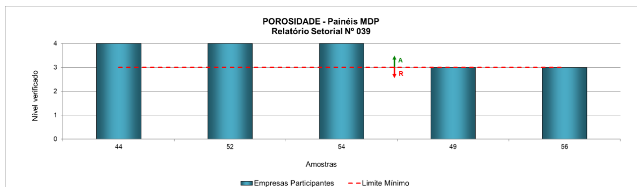
Figura 26 – Porosidade de painéis MDP com revestimento BP, nas duas faces, de 15 mm de espessura
