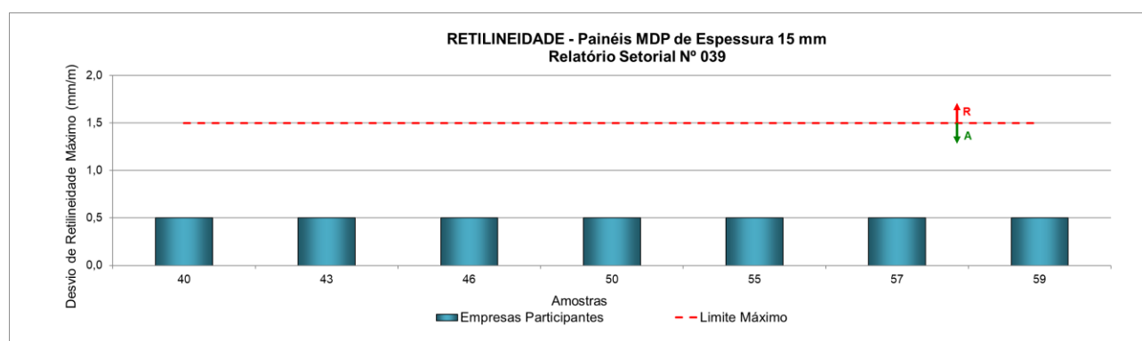
Figura 22 – Desvio de retilidade de painéis MDP sem revestimento de 15 mm de espessura
