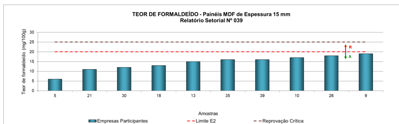
Figura 2 – Teor de formaldeído (método perforator ) de painéis MDF sem revestimento de 15 mm de espessura
