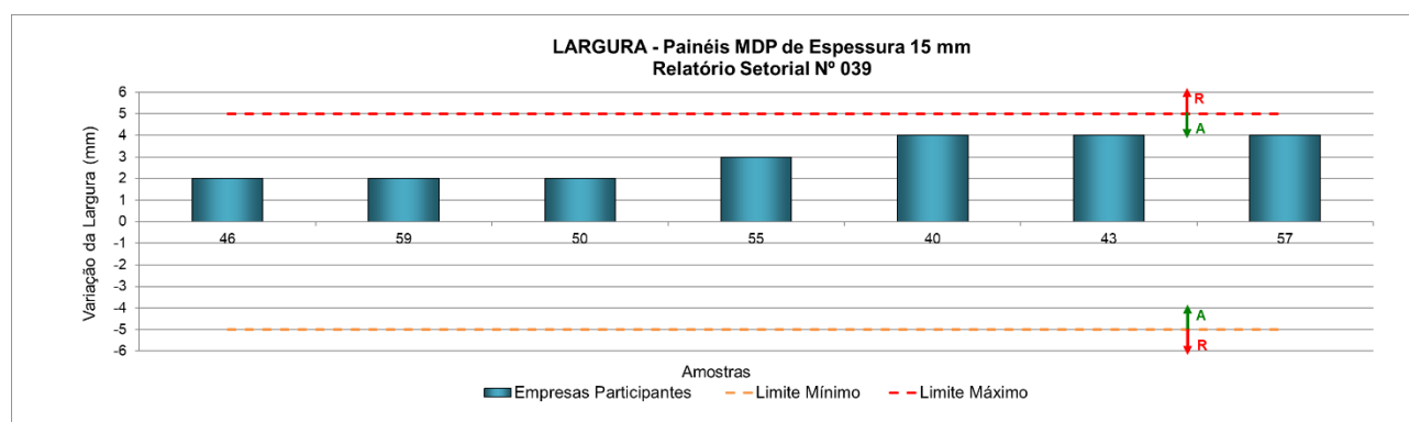
Figura 19 – Variação da largura de painéis MDP sem revestimento de 15 mm de espessura
