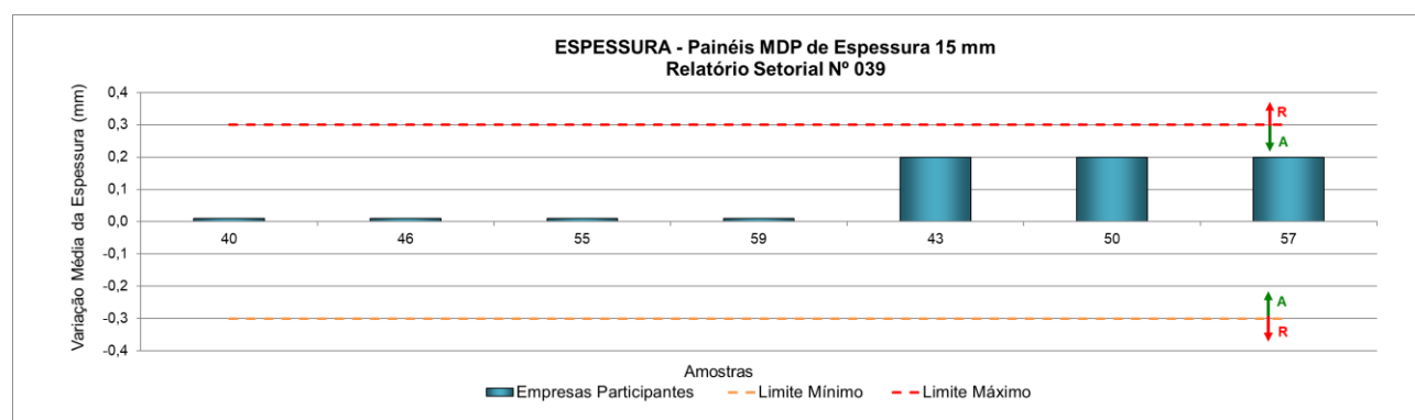
Figura 17 – Variação média da espessura de painéis MDP sem revestimento de 15 mm de espessura
