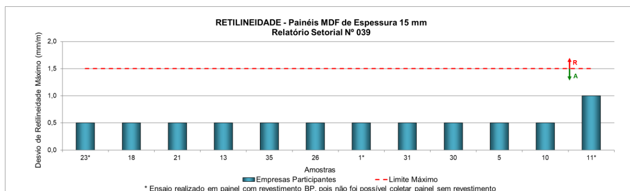
Figura 9 – Desvio de retilidade de painéis MDF sem revestimento de 15 mm de espessura
