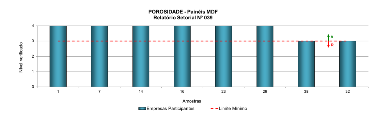
Figura 13 – Porosidade de painéis MDF com revestimento BP, nas duas faces, de 15 mm de espessura
