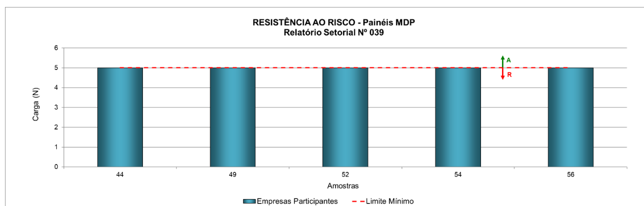
Figura 25 – Resistência ao risco de painéis MDP com revestimento BP, nas duas faces, de 15 mm de espessura
