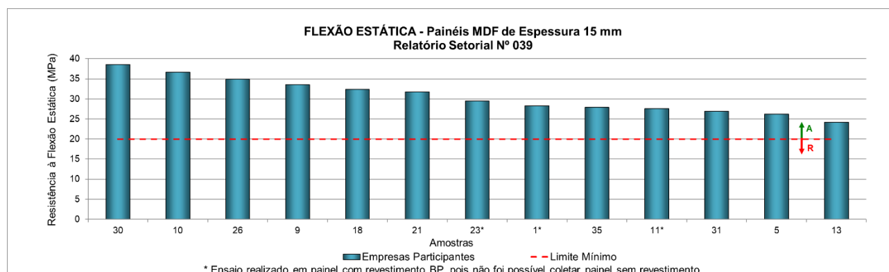
Figura 10 – Resistência à flexão estática de painéis MDF sem revestimento de 15 mm de espessura
