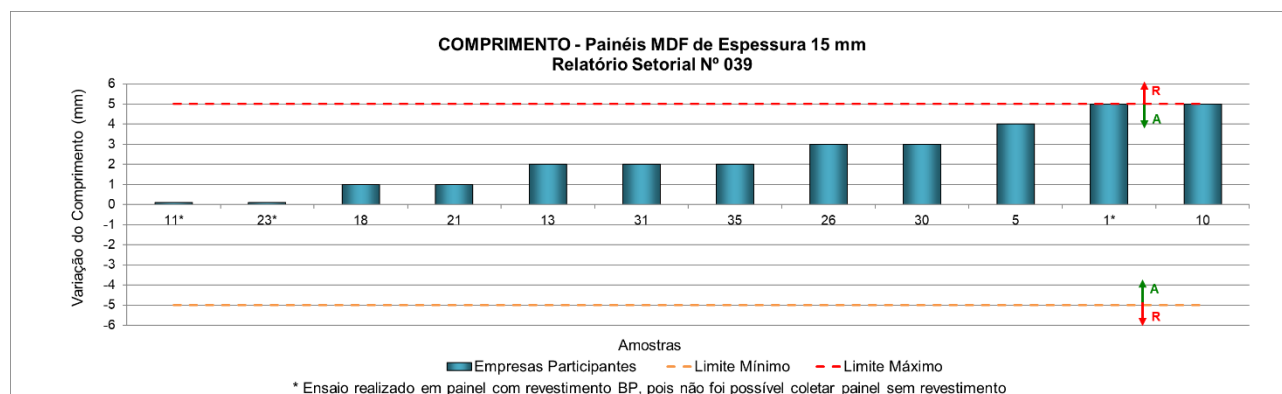
Figura 7 – Variação do comprimento de painéis MDF sem revestimento de 15 mm de espessura
