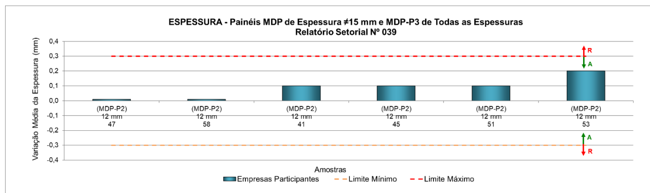
Figura 18 – Variação média da espessura de painéis MDP sem revestimento de espessuras diferentes de 15 mm
