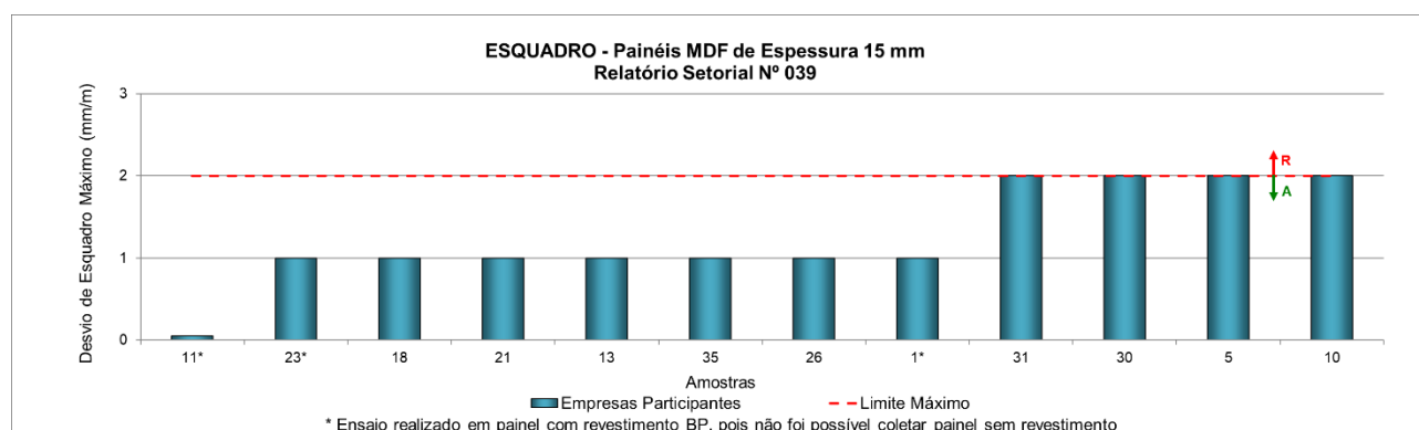
Figura 8 – Desvio de esquadro de painéis MDF sem revestimento de 15 mm de espessura
