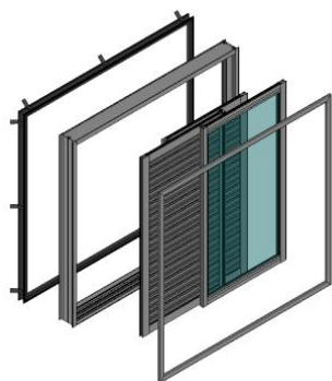
Figura 34 – Instalação da Esquadria (Imagem Cedida Pela AFEAL)
