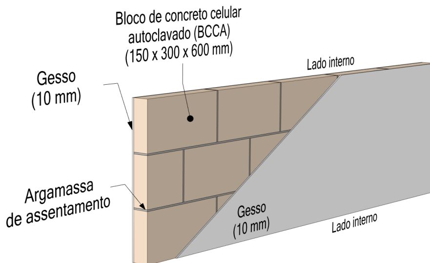
Figura 1 - Esquemas do elemento construtivo, objeto desta FAD, para vedação somente interna
